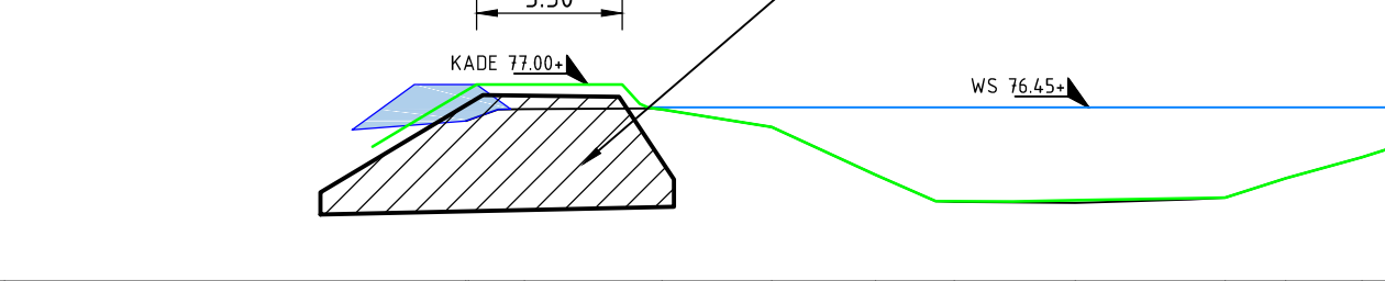
Dwarsprofiel 2 Schaal 1:200
