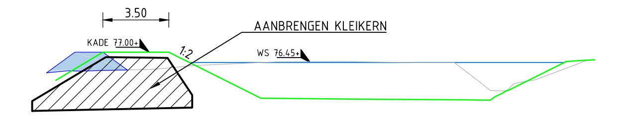
Dwarsprofiel 1 Schaal 1:200
