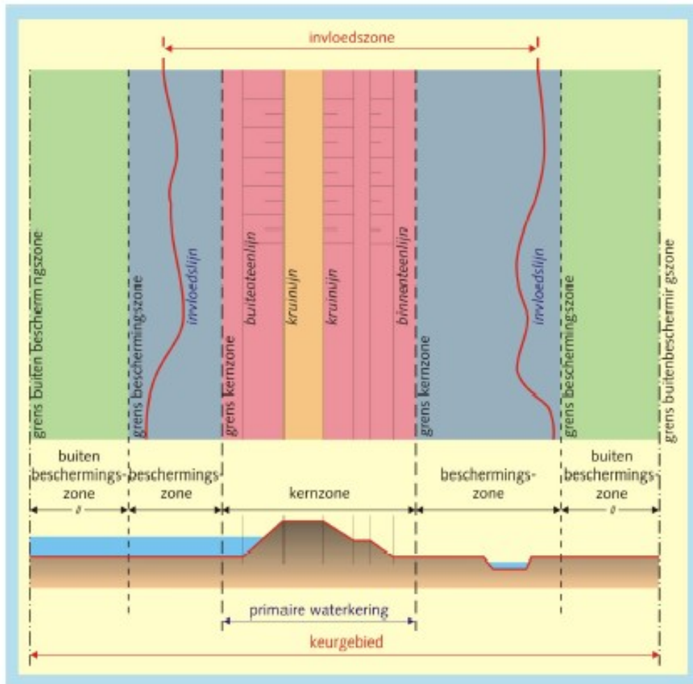
Figuur 1: Benamingen van karakteristieke kenmerken van het dwarsprofiel van een dijk
