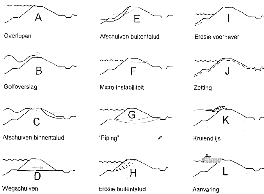
Figuur 2: Overzicht potentiële faalmechanismen
