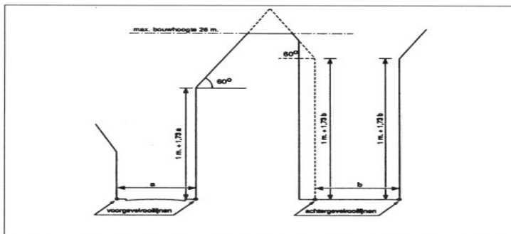
Figuur 14 Bouwhoogte in voor- en achtergevelrooilijn en daartussen. Maximum bouwhoogte (artikelen 2.5.20, 2.5.21, en 2.5.23 en 2.5.24, alternatief 2). Binnen grootstedelijke delen van de bebouwde kom
