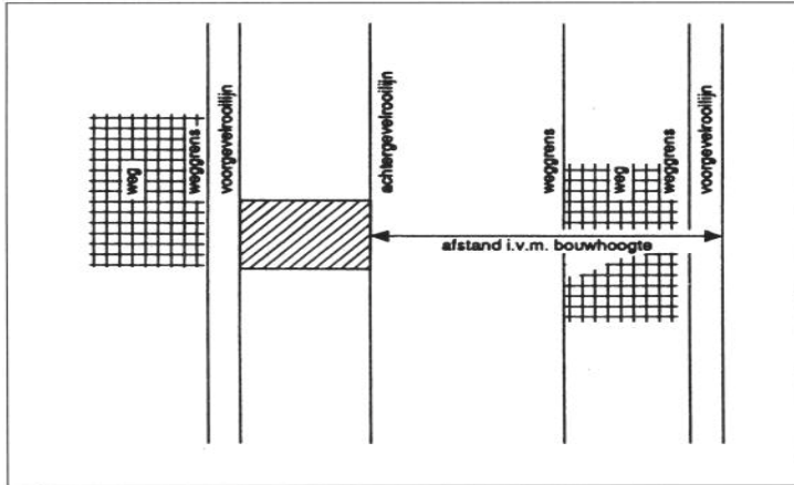
Figuur 18 Bouwhoogte in de achtergevelrooilijn (2.5.20, tweede lid, tweede alinea)
