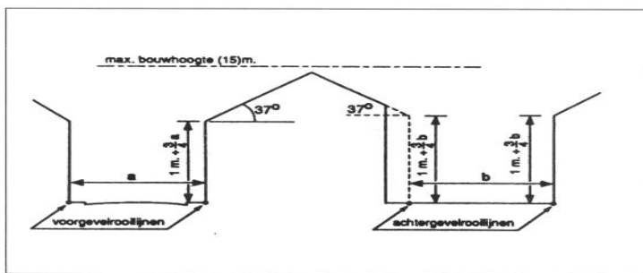
Figuur 13 Bouwhoogte in voor- en achtergevelrooilijn en daartussen. Maximum bouwhoogte (artikelen 2.5.20, 2.5.21, 2.5.23 en 2.5.25). Buiten de bebouwde kom
