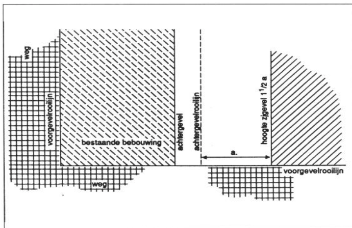
Figuur 18 Bouwhoogte in de achtergevelrooilijn (2.5.20, tweede lid, tweede alinea)
