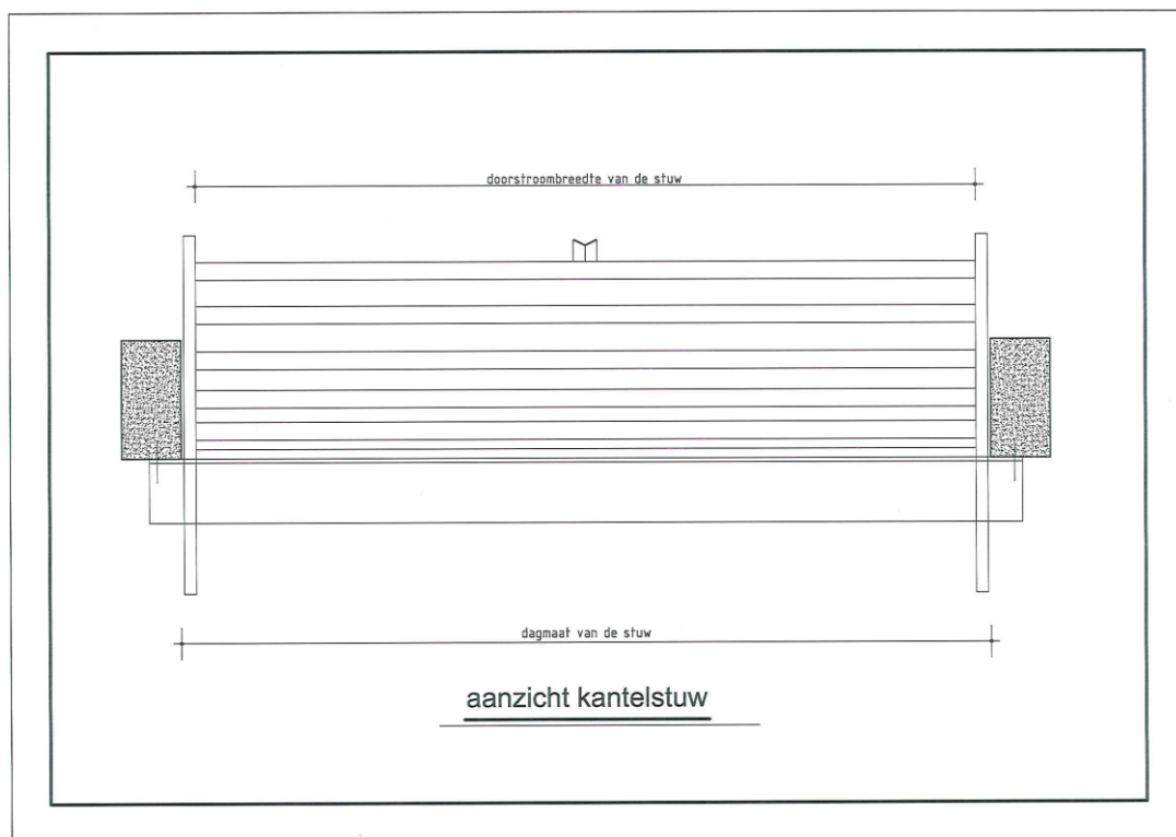
Technische tekening met zij- en vooraanzicht van een kantelstuw
