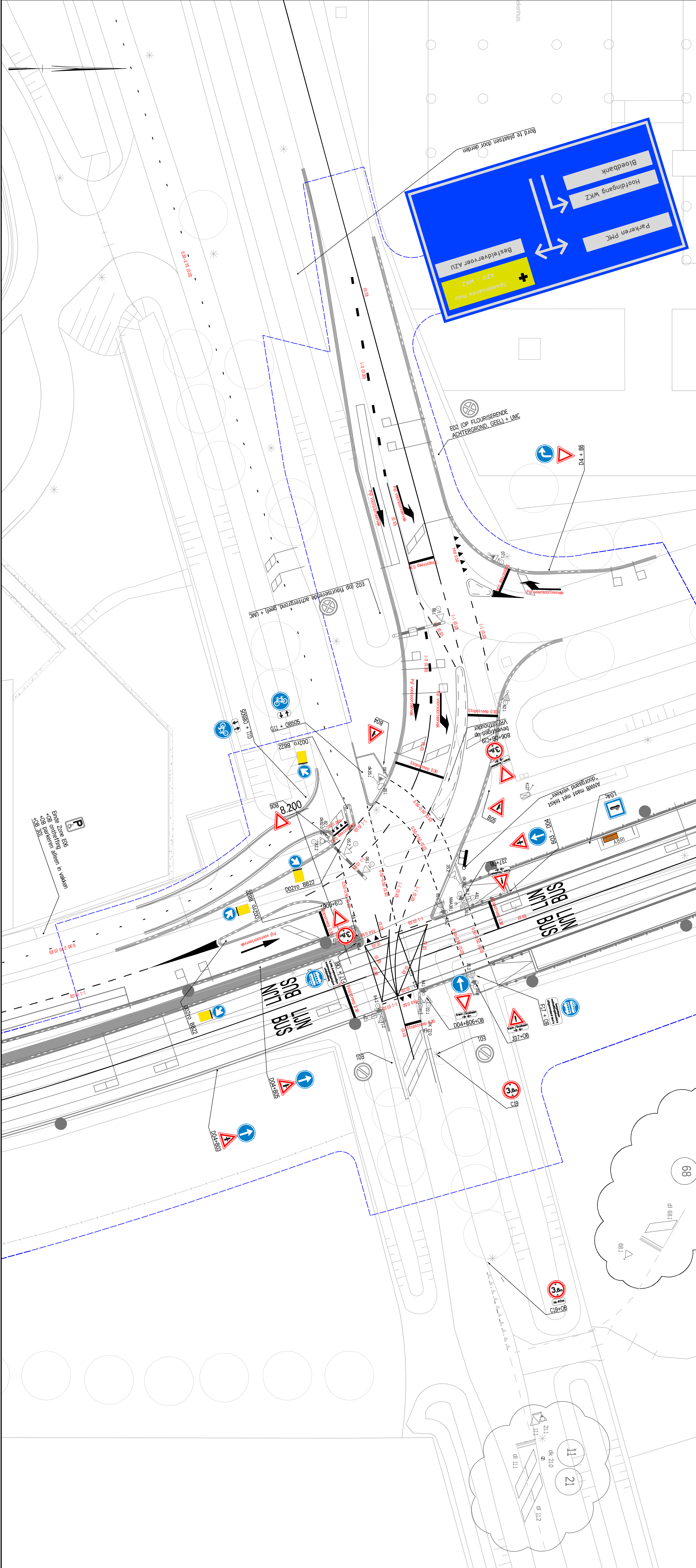
Situatie kruising hoofdrij
