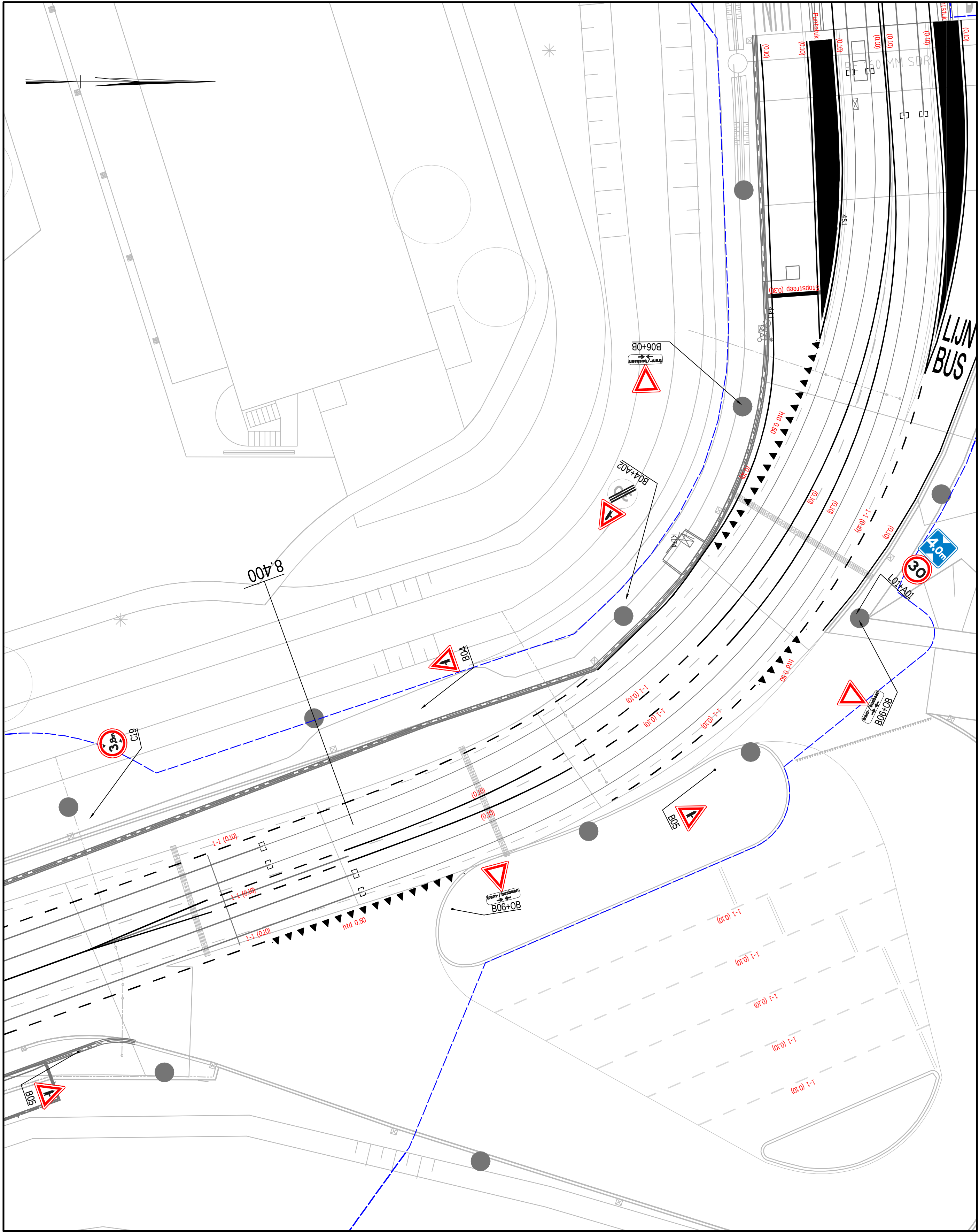
Situatie kruising WKZ
