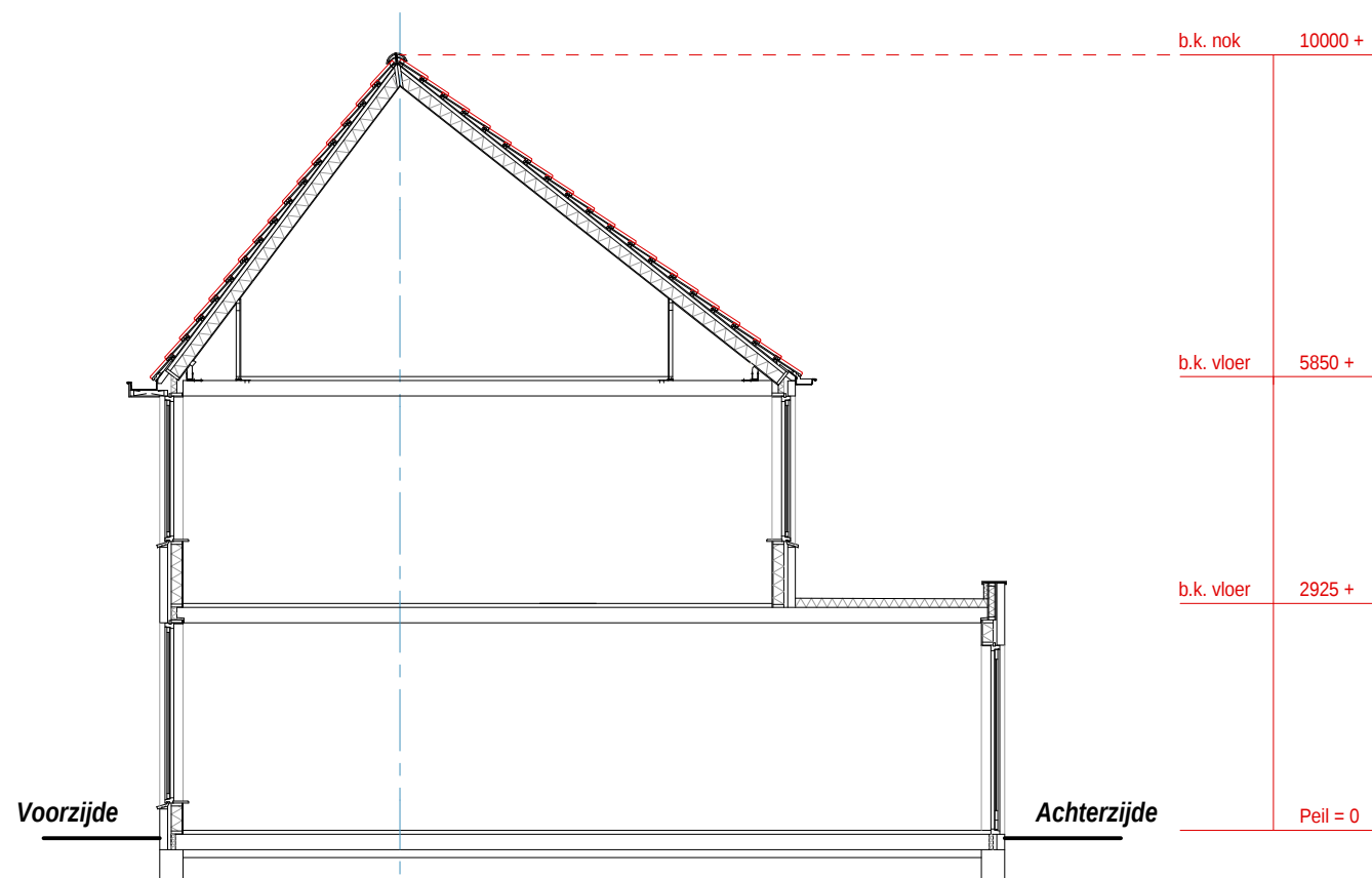
Doorsnede Bestaand
