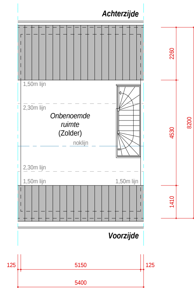
Zolderverdieping Bestaand
