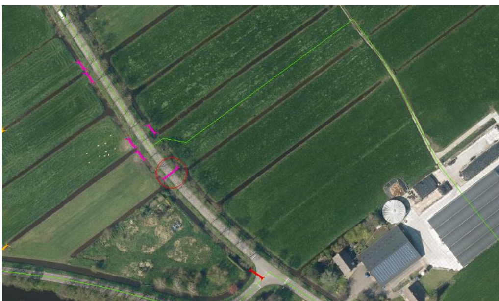
Figuur 6.3: ligging te vervangen duiker Hoogendoornlaan
