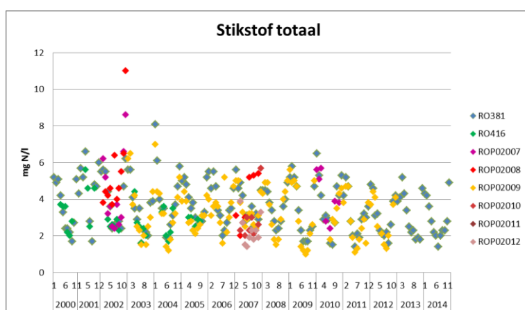
Figuur 4-4: Meetwaarden stikstof totaal (RO = meetpunt boezem, ROP = meetpunt polder)
