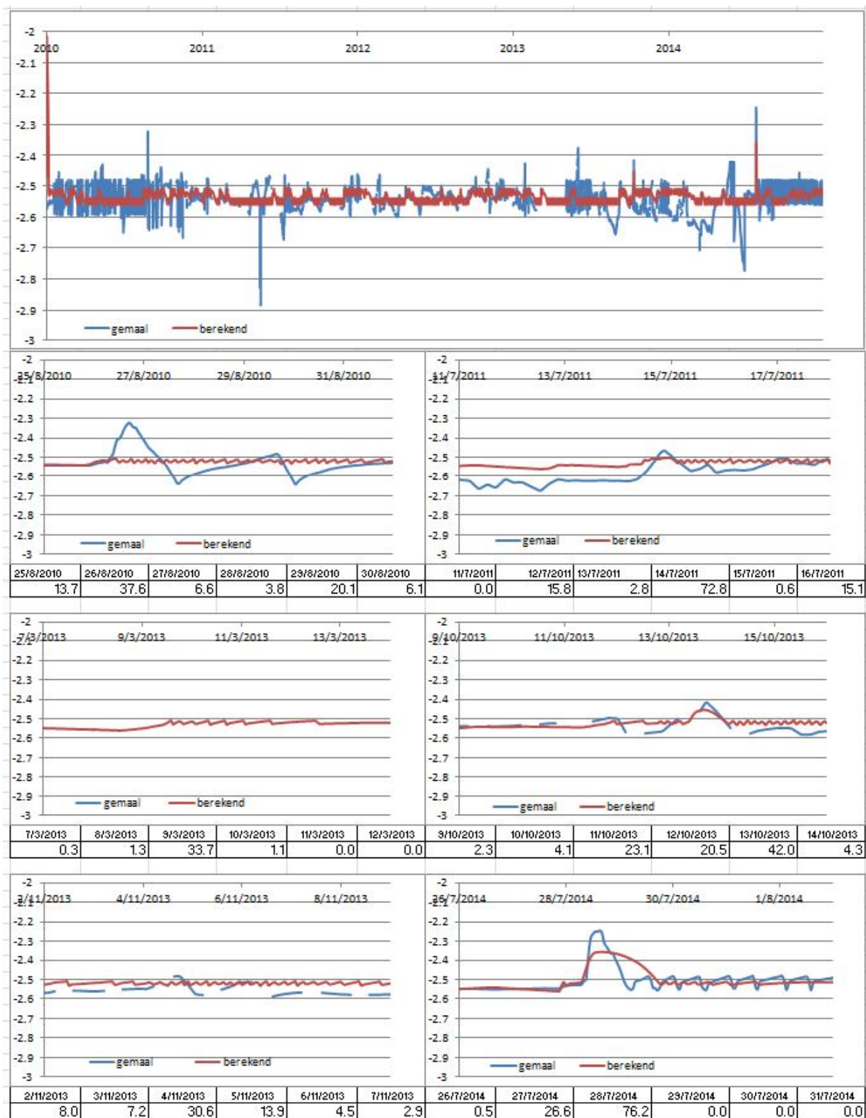
Figuur 7 : Berekende en gemeten waterstanden (bij gemaal) voor peilvak WW-42C
