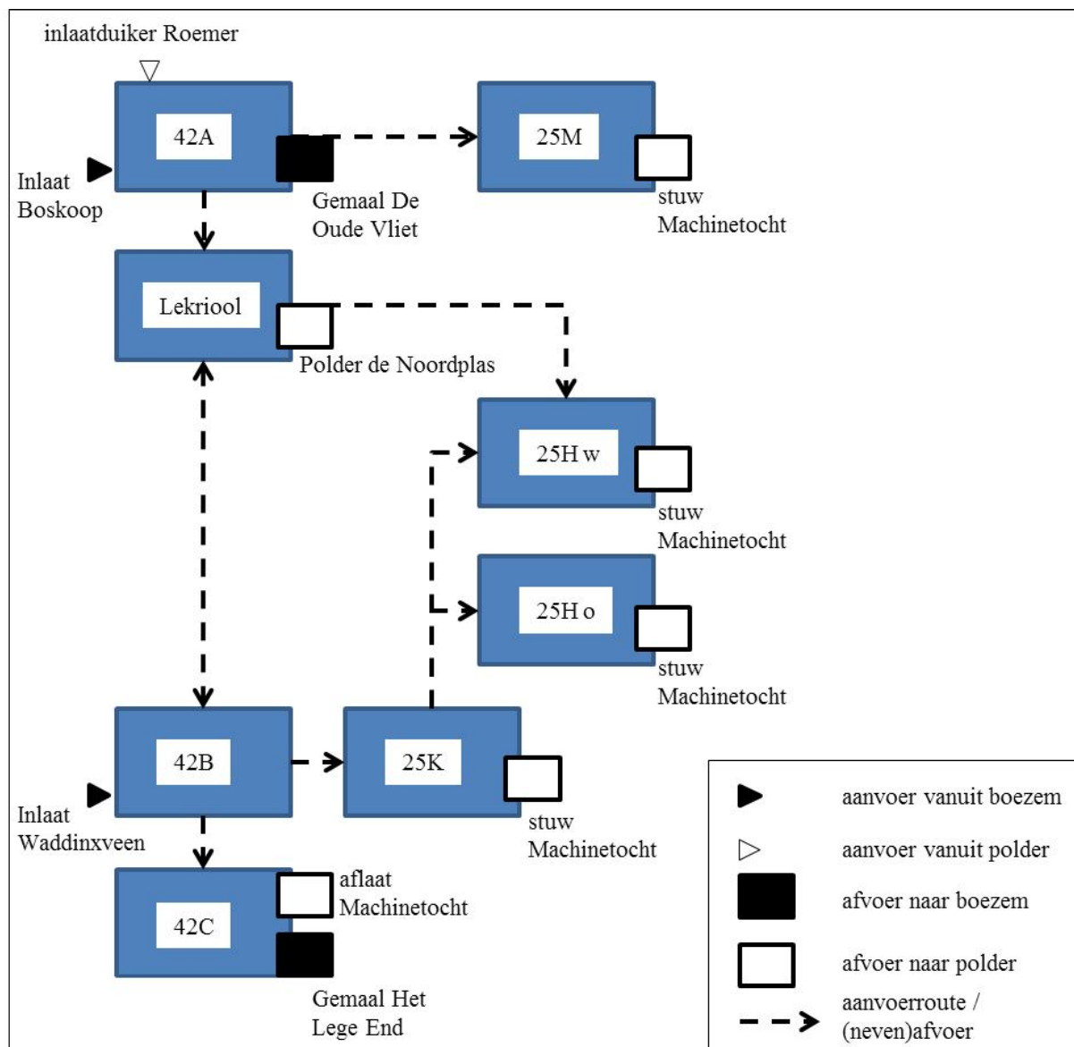
Figuur 4-1: Schematisch overzicht wateraanvoer en -afvoer peilbesluitgebied Voorofse Polder e.o.
