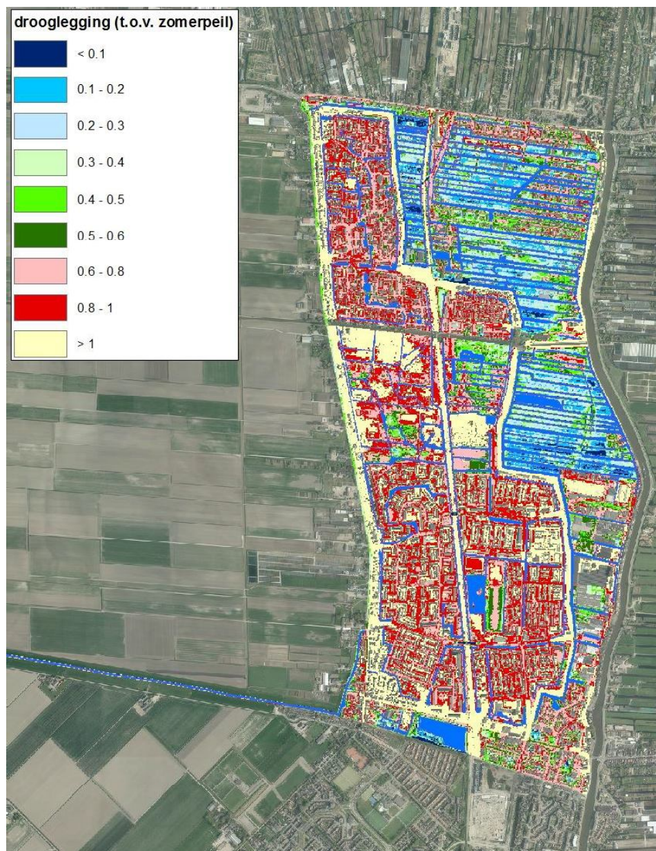
Figuur 2: Drooglegging t.o.v. zomerpeil
