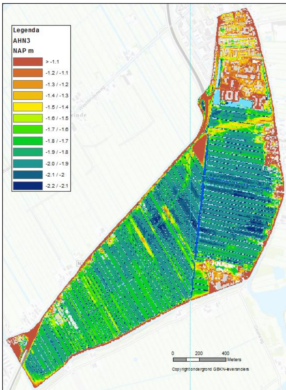
Figuur 3-5 Maaiveldhoogte (m NAP) in de Zwet- en Grote Blankaartpolder.
