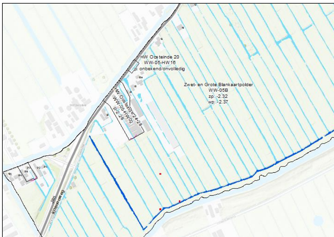
Figuur 4-2 Inundatiekaartje zuiden van Zwet- en Grote Blankaartpolder. Inundatie is rood gemarkeerd weergegeven.
