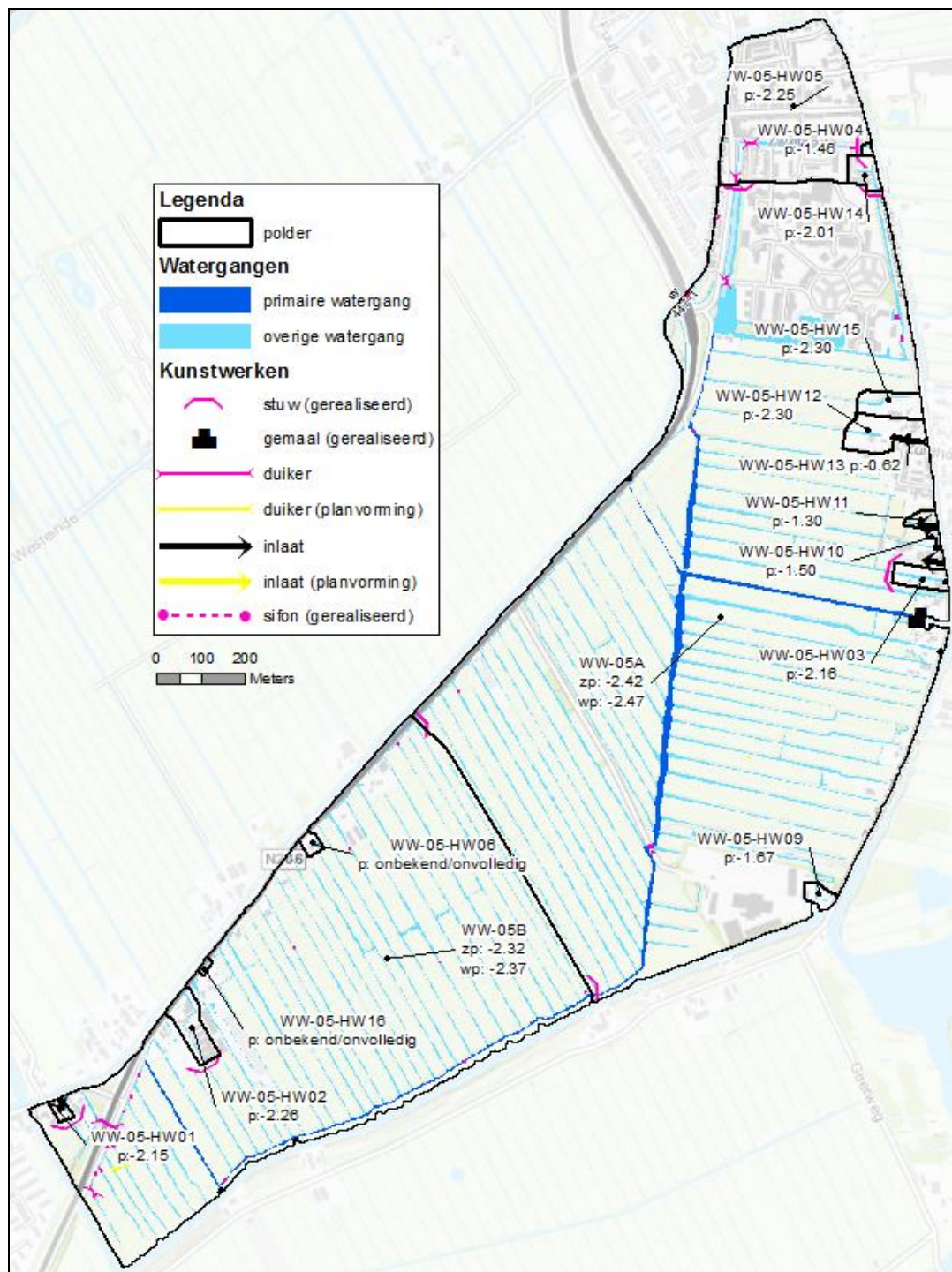
Figuur 3-7 Watersysteemkaart Zwet- en Grote Blankaartpolder
