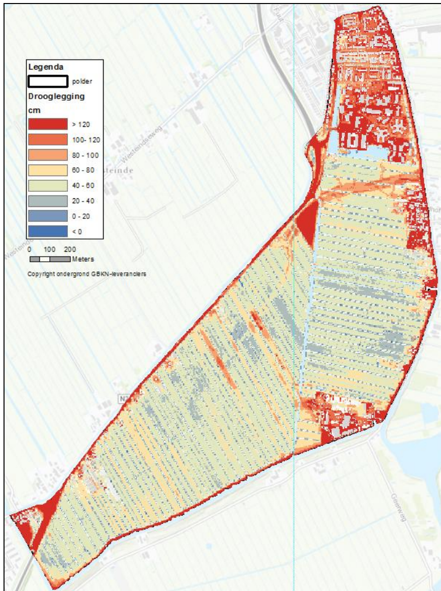
Figuur 4-4 Drooglegging Grote Zwet- en Blankaartpolder bij zomerpeil
