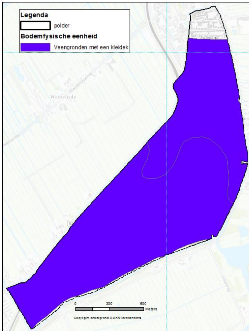
Figuur 3-4 Bodemkaart (Stiboka, 1966)
