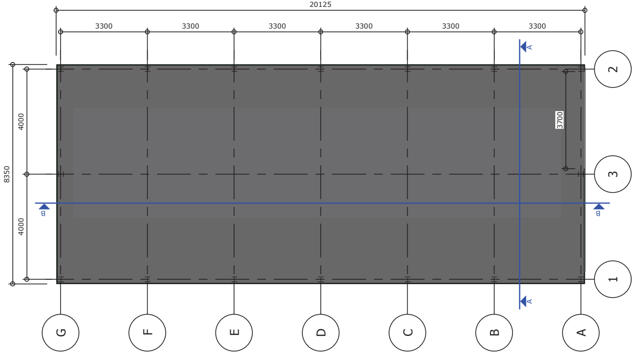
Plattegrond 1:100
