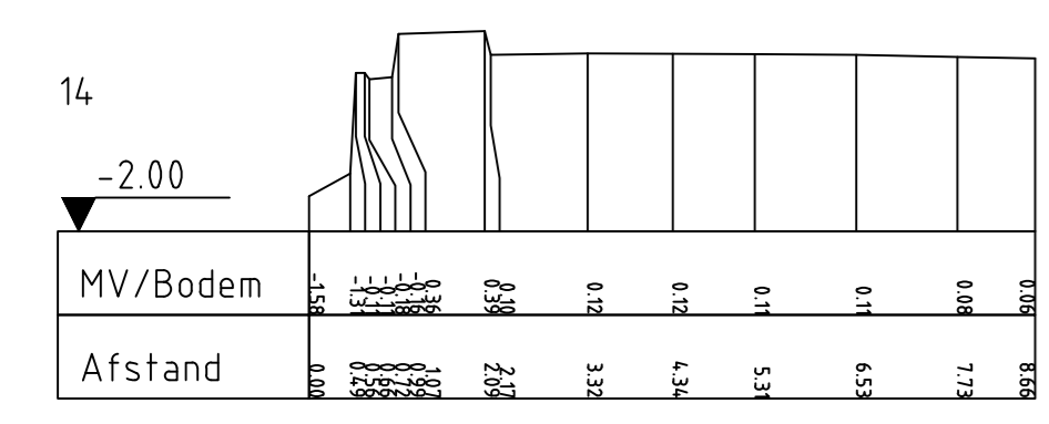
INGEMETEN DWARSPROFIELEN
