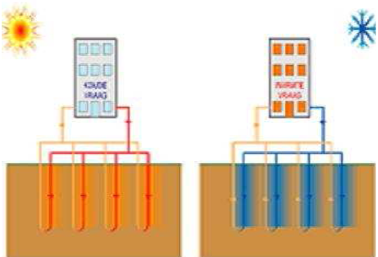
Afbeelding 2. Gesloten bodemenergiesysteem
