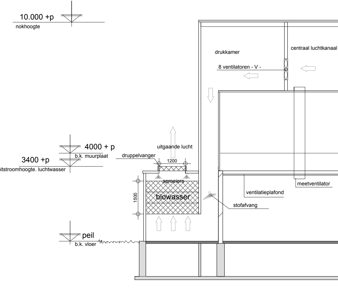
Doorsnede Luchtwasser BWL 2009.12.V2 stal 4 1800 vleesvarkens + 600 gesp. biggen
