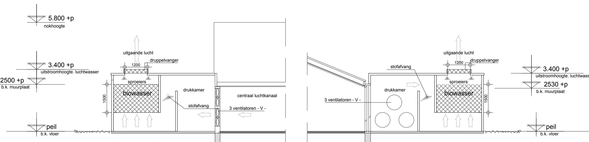
Doorsnede Luchtwasser BWL 2009.12.V2 stal 1 588 vleesvarkens
