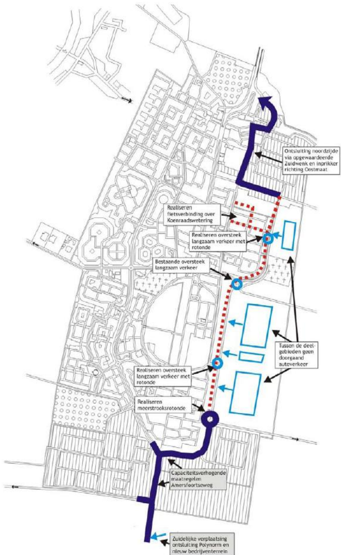
Figuur 12 Aanpassingen hoofdwegen oostzijde
