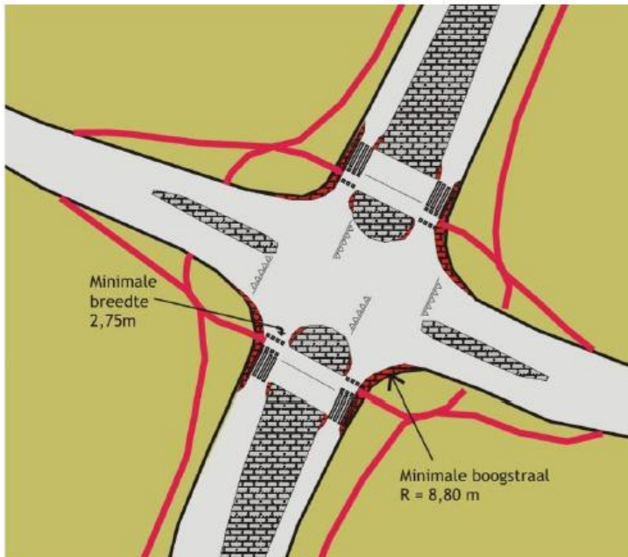
Figuur 9 Principeoplossing voor versmalling ter hoogte van de oversteek voor fietser en voetganger
