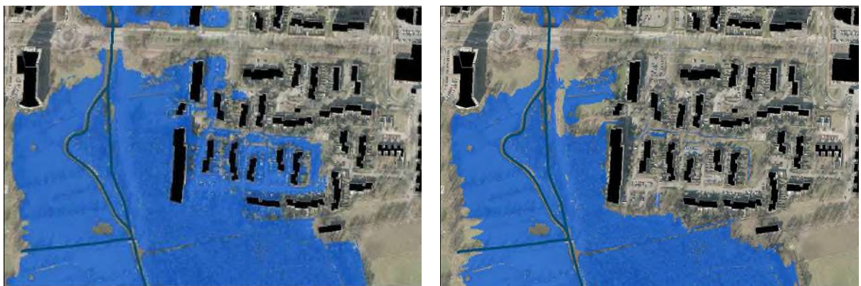
Figuur 5-28 Inundatie Coevering bij T100 W+ in de referentiesituatie (links) en bij T100W+ met inzet waterberging (rechts), gevisualiseerd over het hoogtekart (bron: AHN2 0,5*0,5 m)
