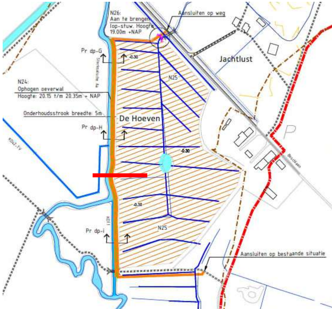
Figuur 3-11 Globale aanduiding (rood) van de locatie van de hieronder getekende dwarsdoorsnede
