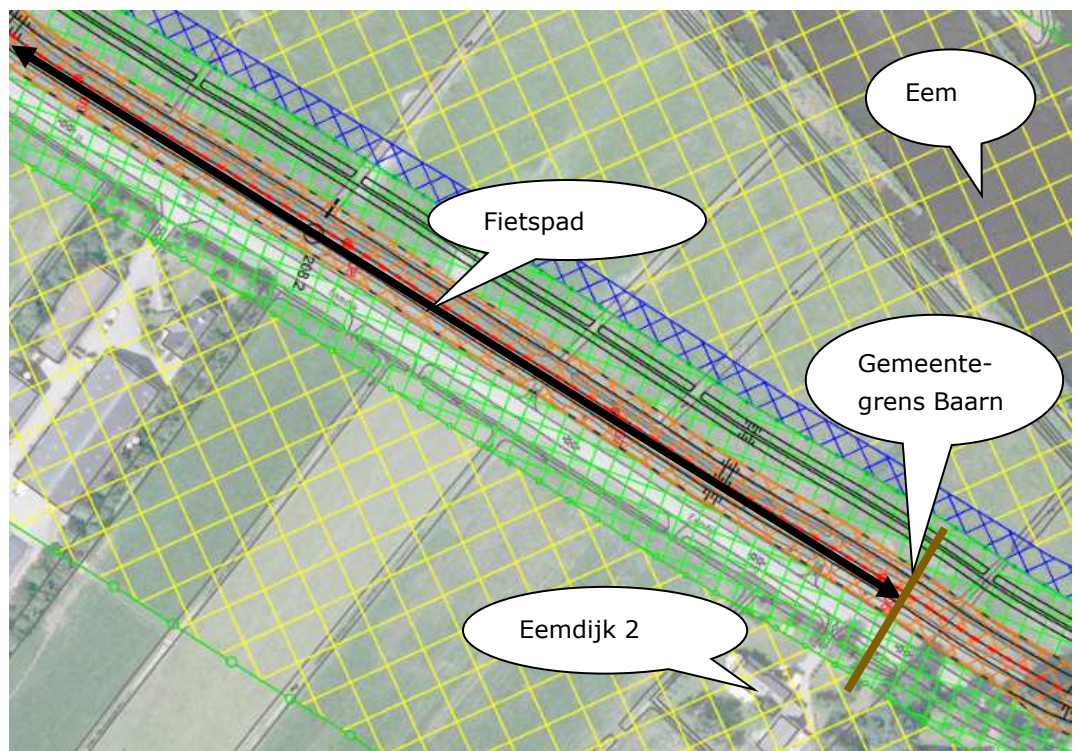
Situatietekening 2:
