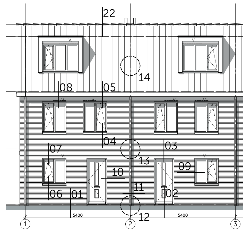
Voorgevel
