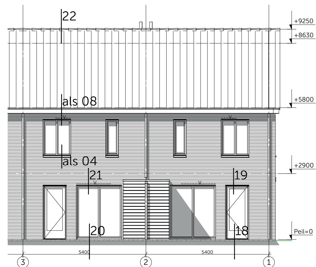
Achtergevel
