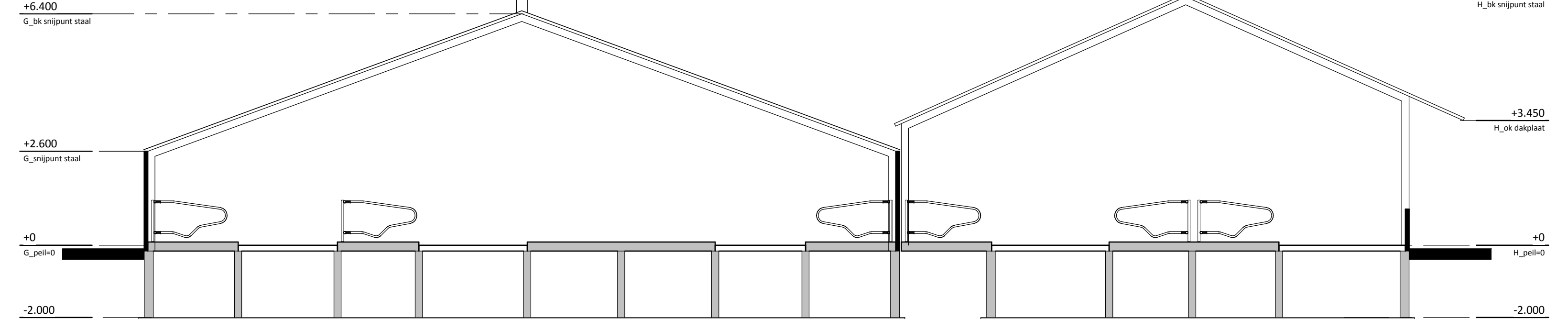
doorsnede G
