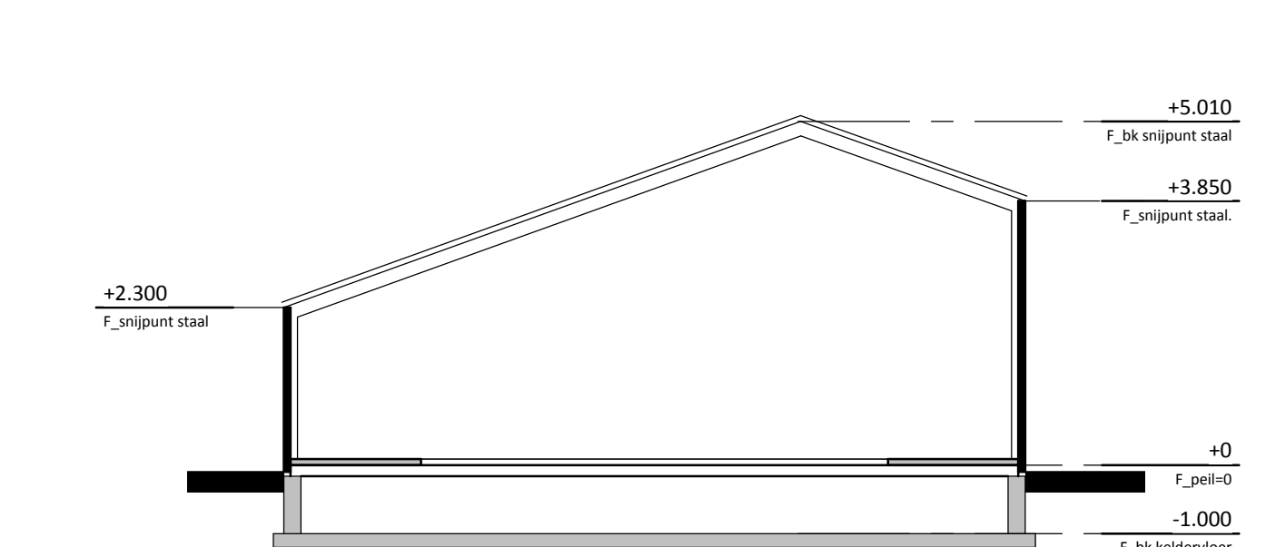
doorsnede DE
