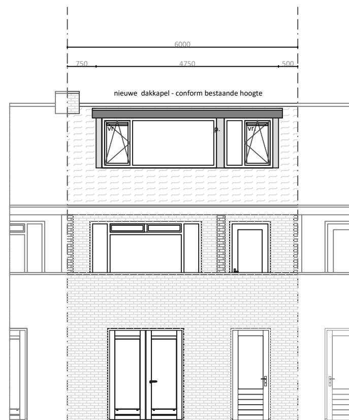
Achtergevel - nieuw
