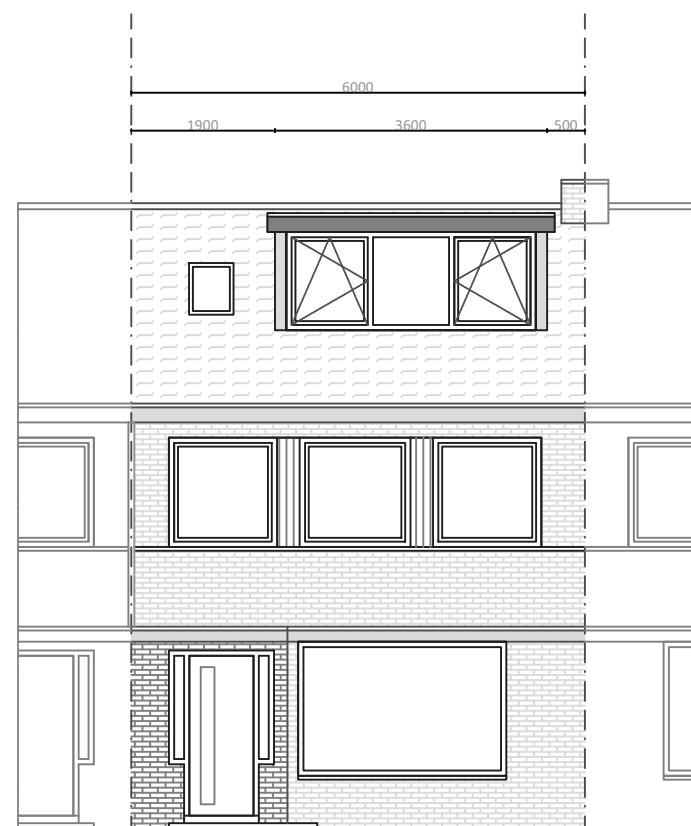
Vorgevel - nieuw
