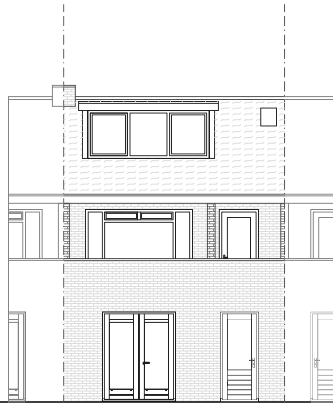
Achtergevel - bestaand
