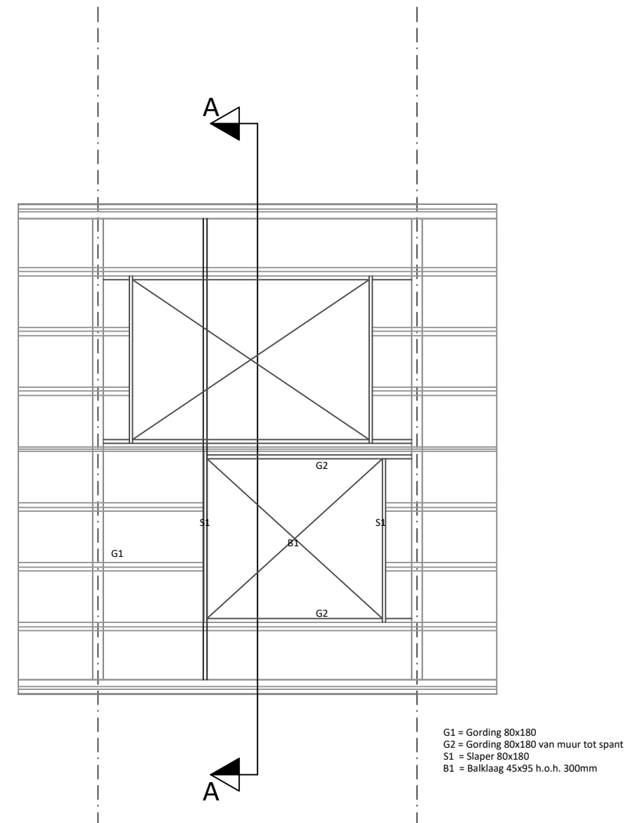
Kapplan - nieuw
