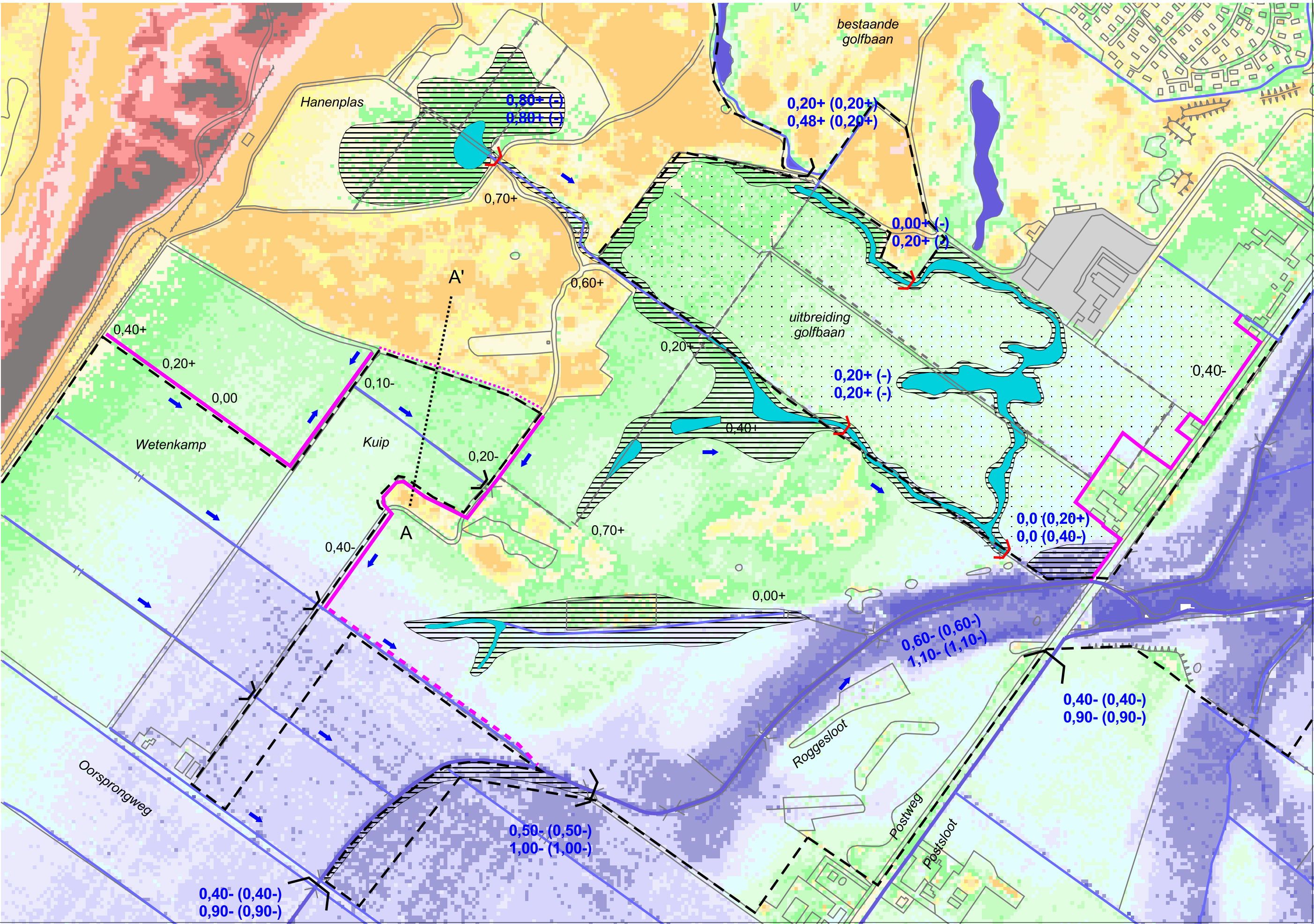
Voorstel waterhuishoudkundige afstemming Hanenplas - agrarische omgeving
