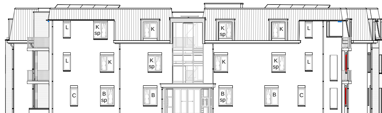
Rechter zijgevel:
