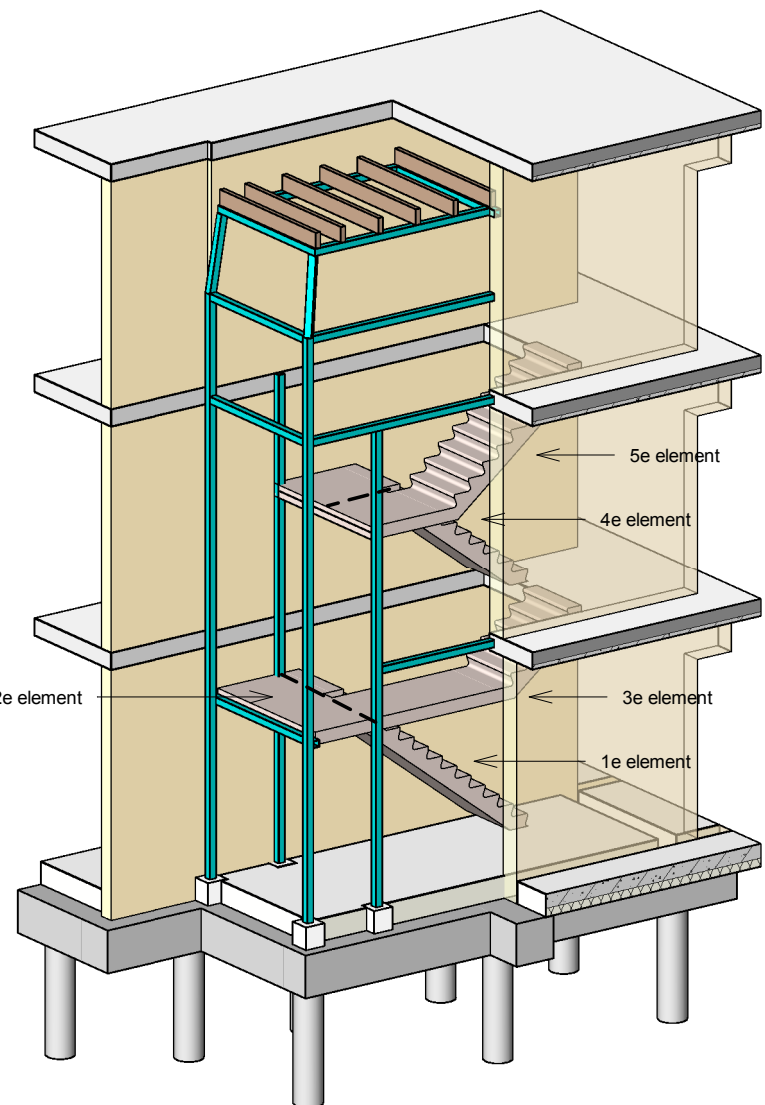
3D - constructie trappenhuis incl. prefabtrappen
