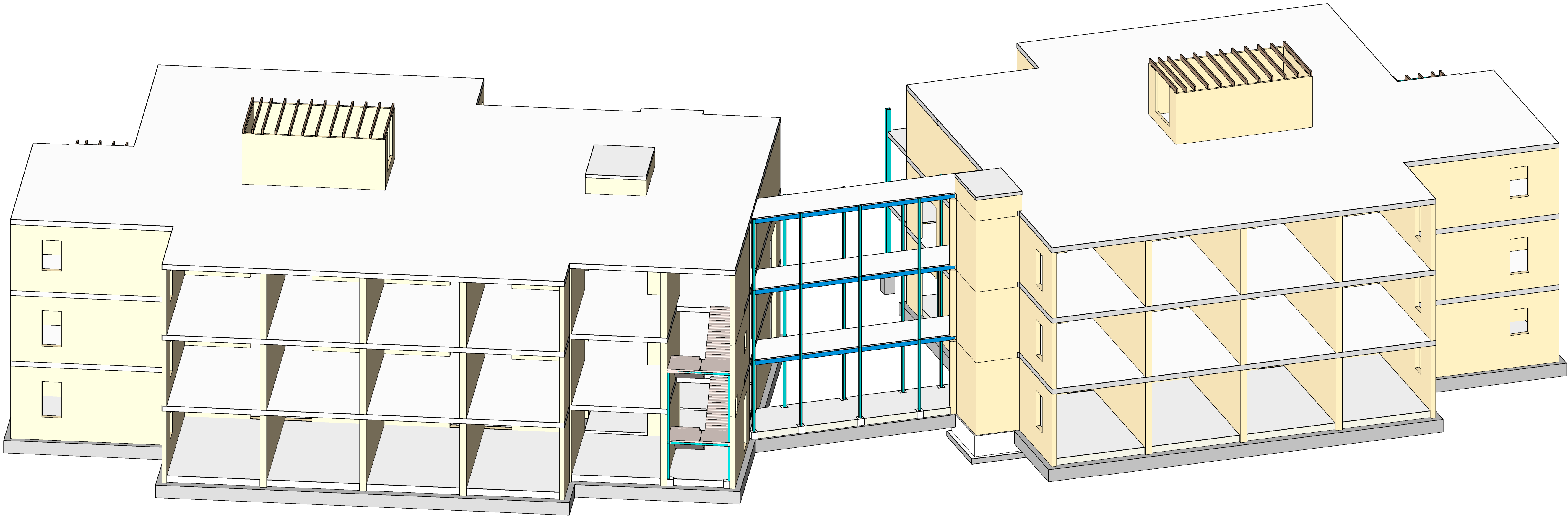
3D - constructie
