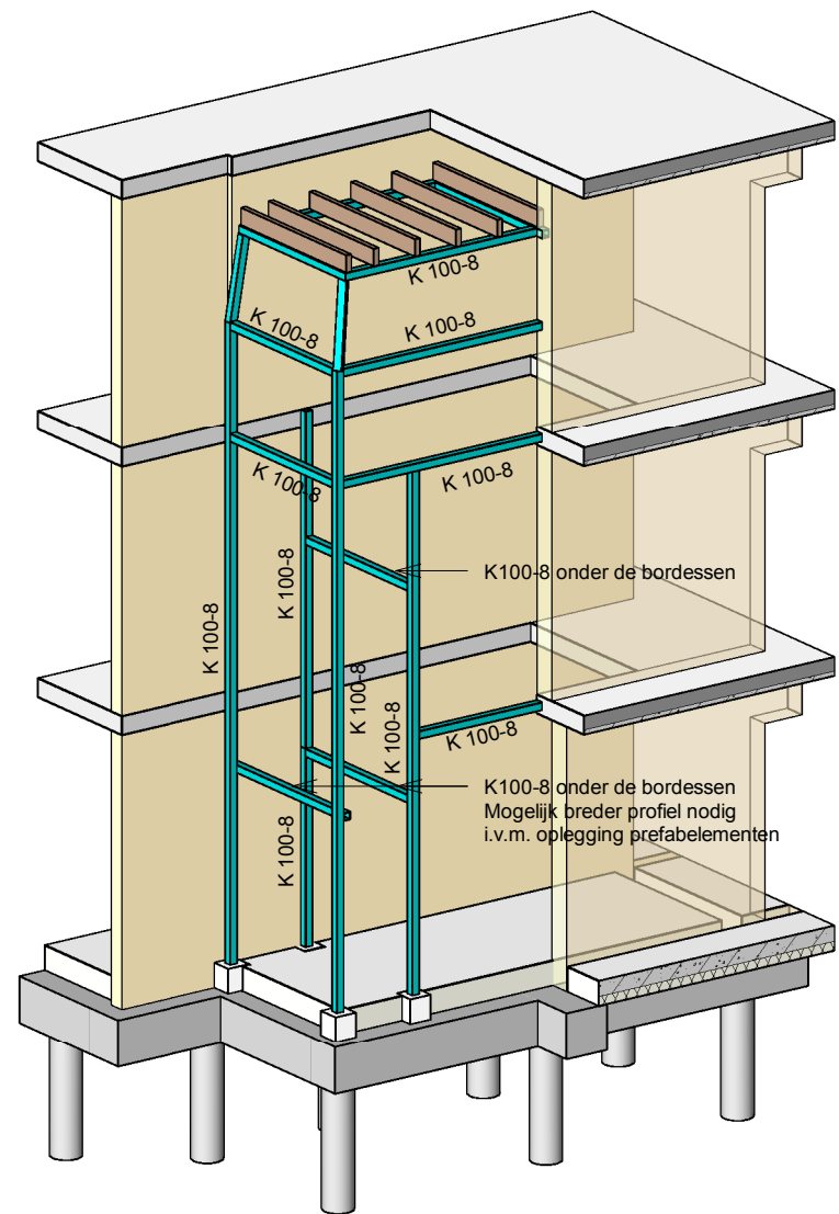
3D - constructie trappenhuis
