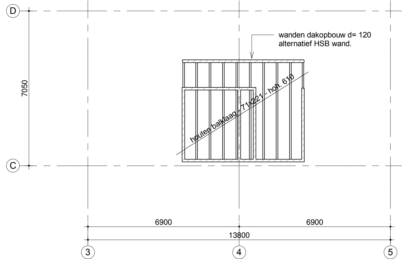
Dakopbouw 1 : 100
