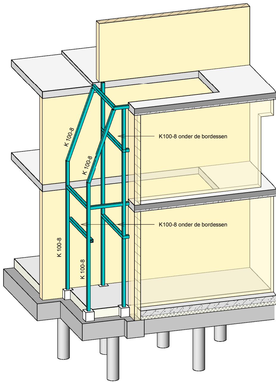
3D - constructie trappenhuis
