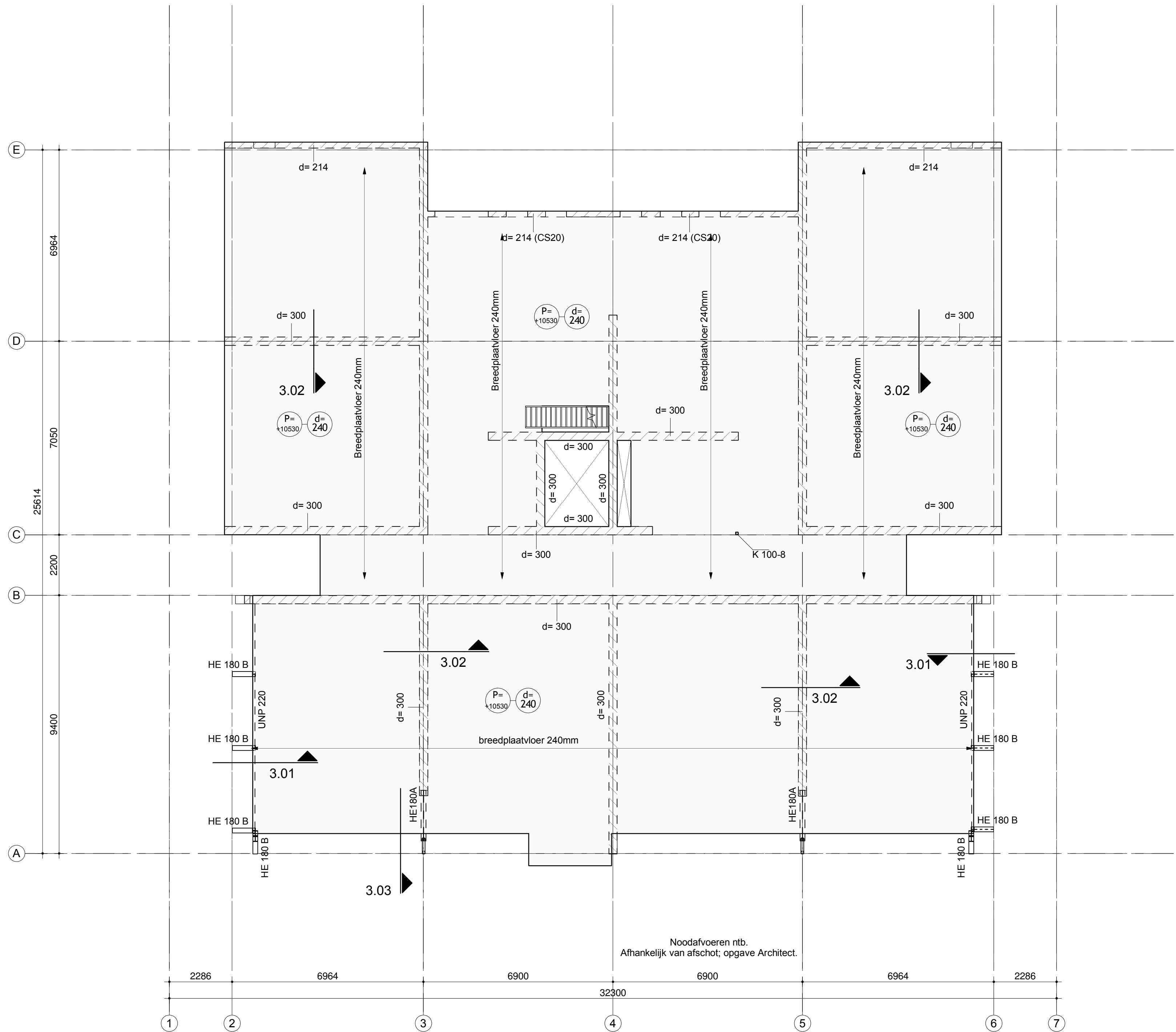
Dak 1 : 100
