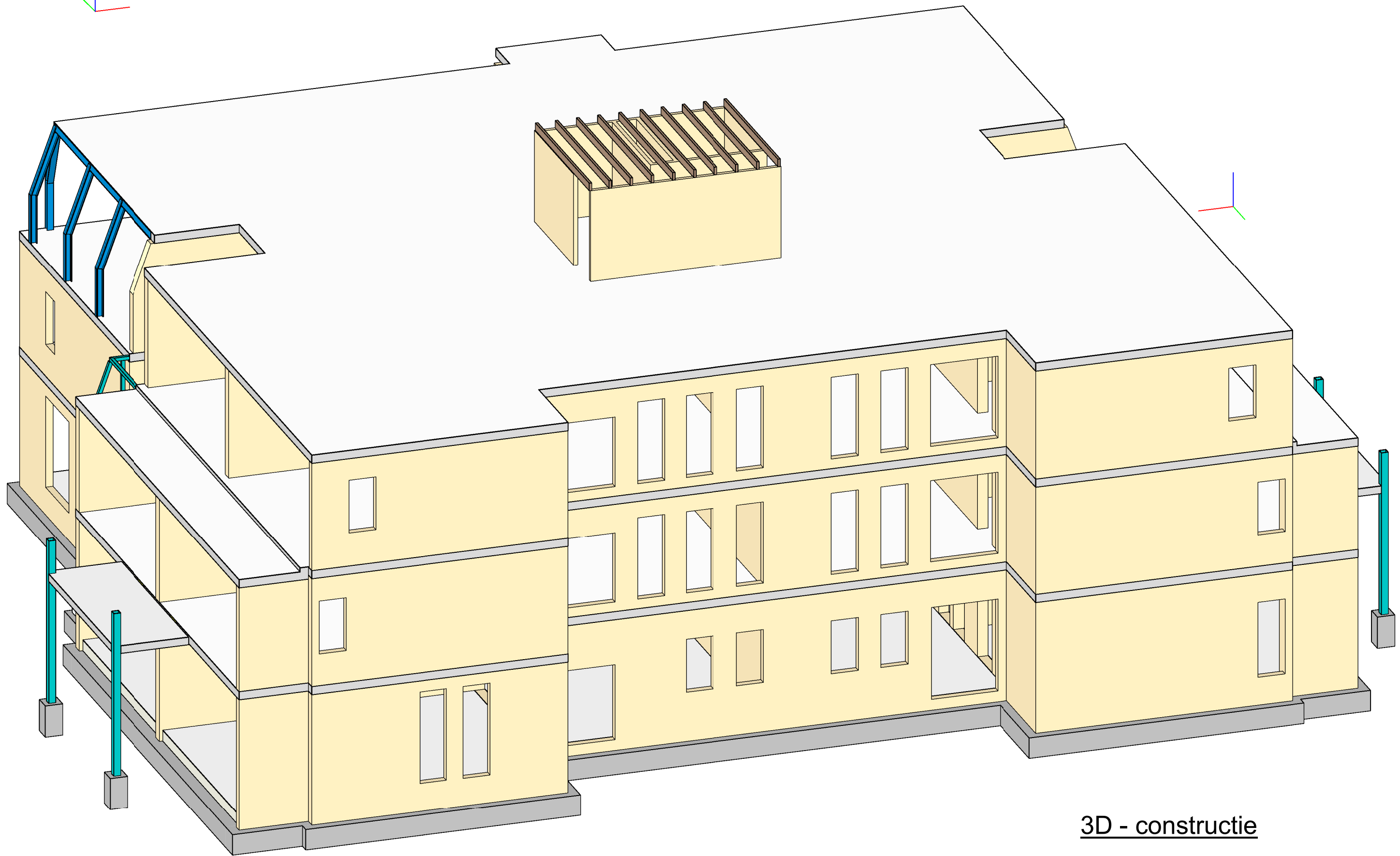
3D - constructie
