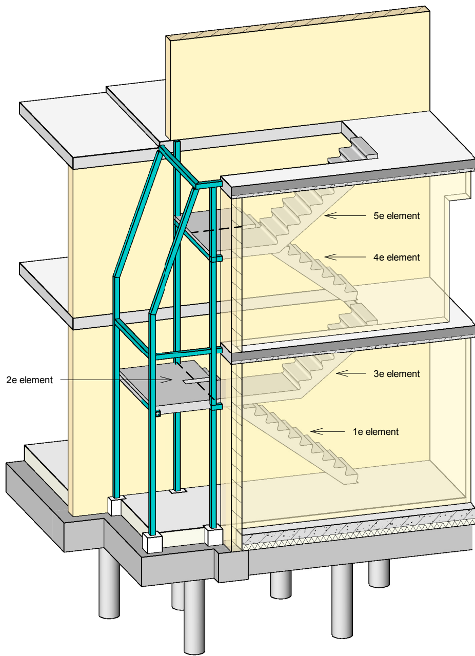
3D - constructie trappenhuis incl. prefabtrappen
