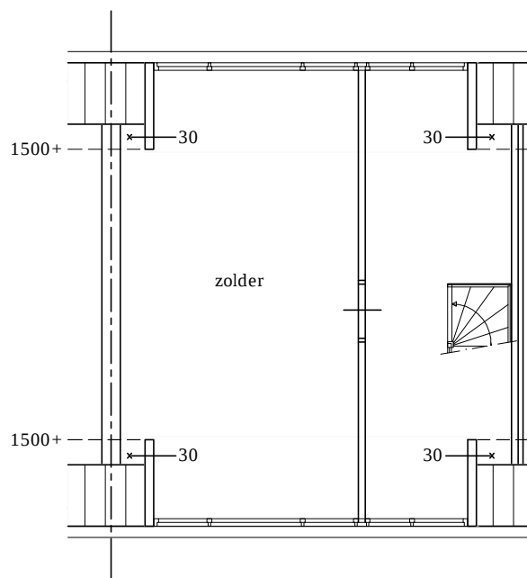
GEWIJZIGDE 2e VERDIEPING
