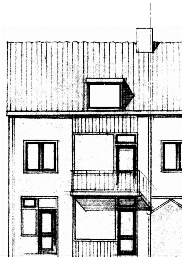
BESTAANDE ACHTERGEVEL
