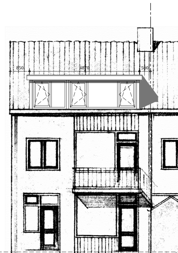
GEWIJZIGDE ACHTERGEVEL
