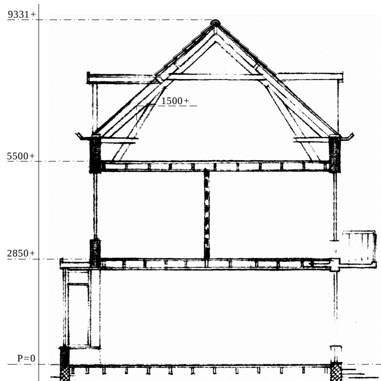
BESTAANDE DOORSNEDE
