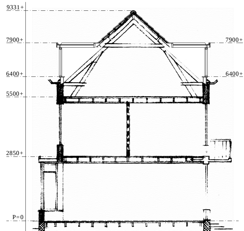
GEWIJZIGDE DOORSNEDE
