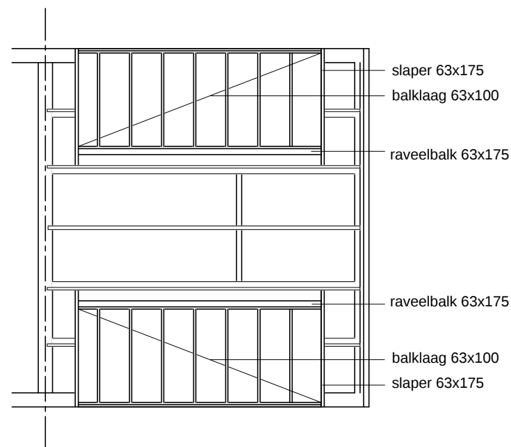
KAPPLAN
