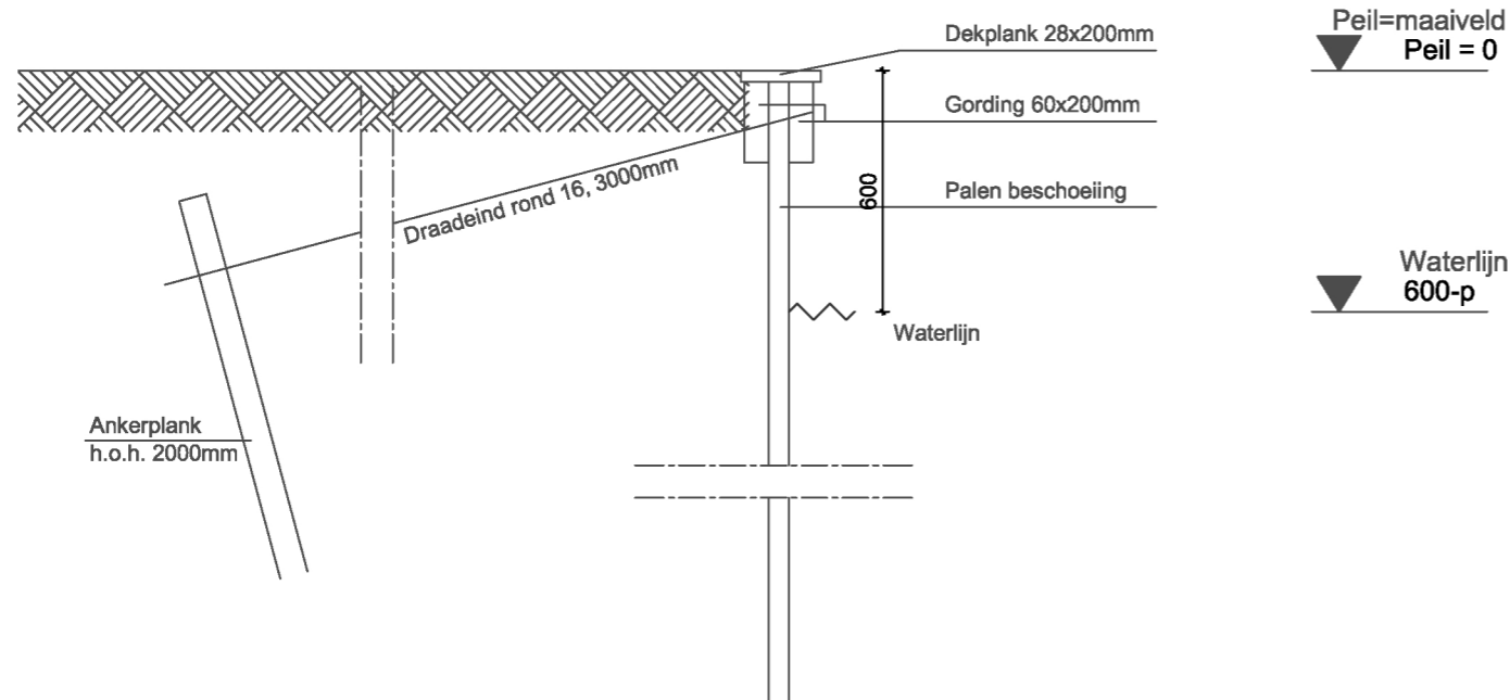
Dwarsdoorsnede 1:20 Bestaand
