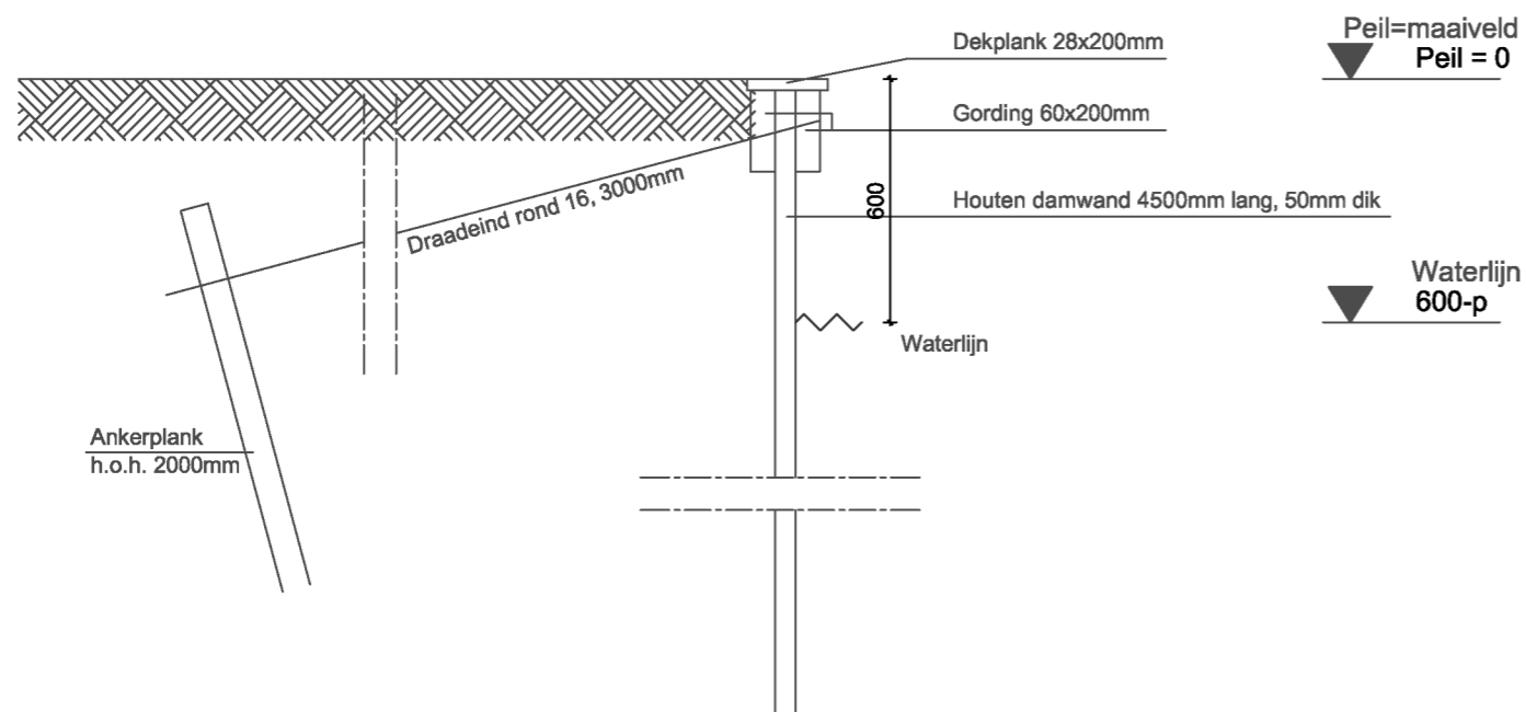
Dwarsdoorsnede 1:20 Nieuw
