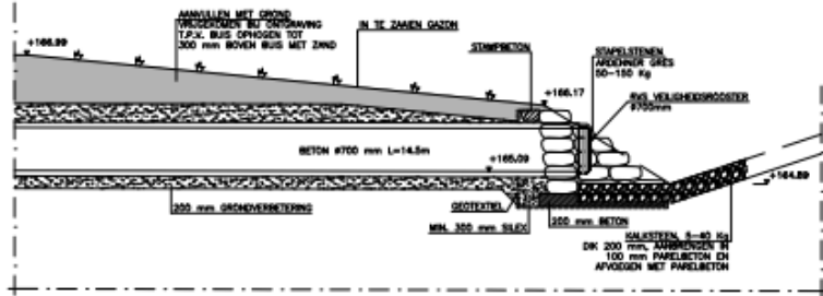
DETAIL 1 DOORENDE UITSTROOMCONSTRUCTIE SCHAL 1:50
