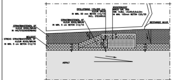
PRINCIPE DETAIL VOORZICHTIG UITSTROOMVOORZIEIING SCHAL 1:50
