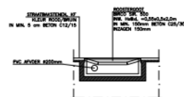
PRINCIPE DETAIL LANGSDOORSNEDIG UITSTROOMVOORZIEIING SCHAL 1:50
