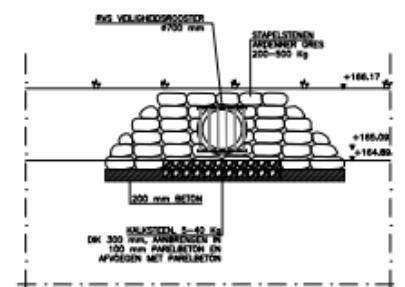
PRINCIPE DETAIL VOORZICHTIG UITSTROOMVOORZIEIING SCHAL 1:50
