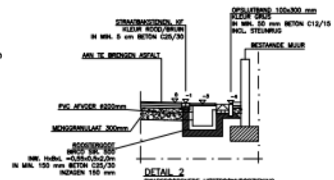
PRINCIPE DETAIL LANGSDOORSNEDIG UITSTROOMVOORZIEIING SCHAL 1:50
