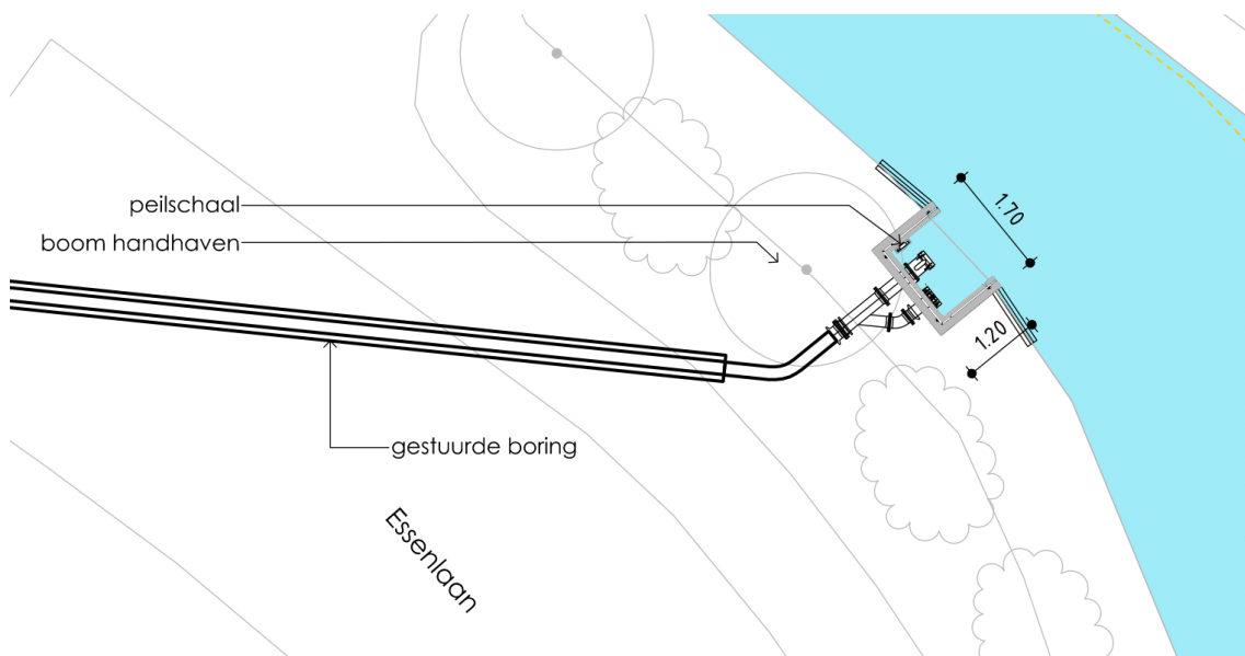
Figuur 7: Bovenaanzicht uitstroomvoorziening Essenlaan
