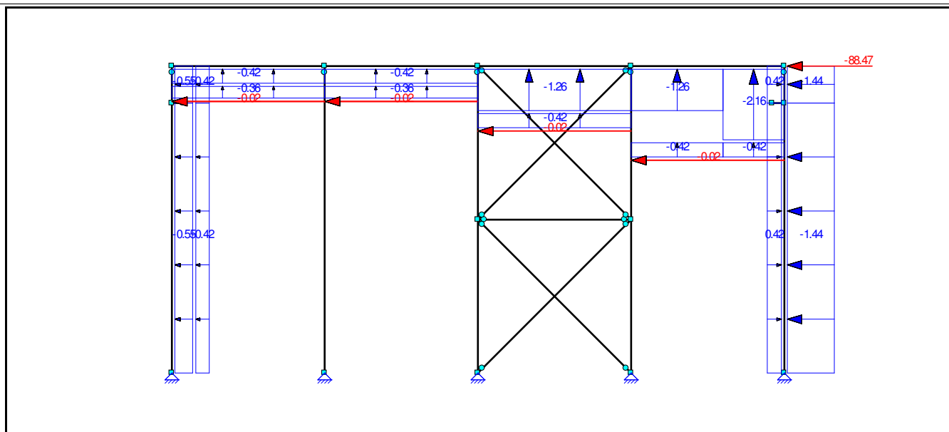
B.G.12: WINDBELASTING VAN RECHTS + OVERDRUK (2E CPE)
