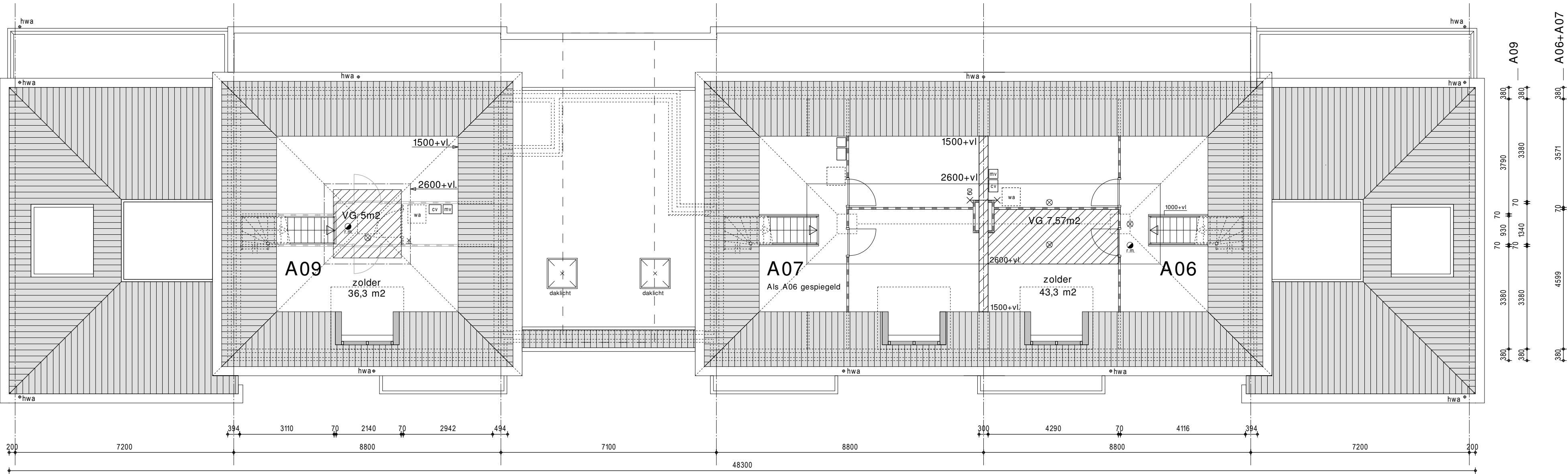
2e verdieping blok A
