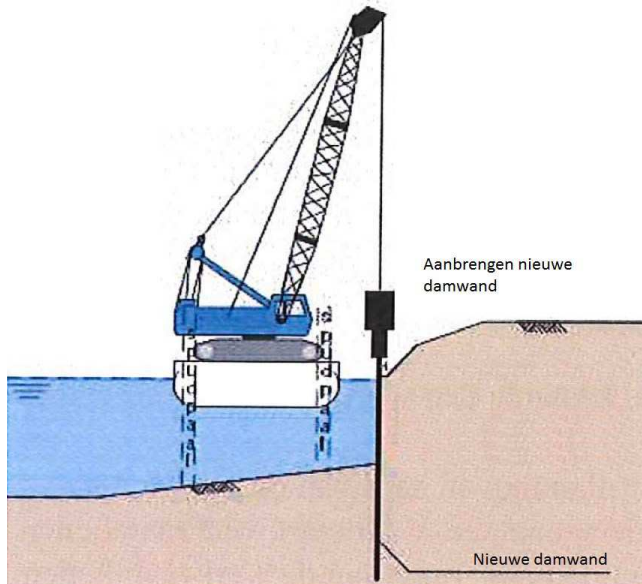
Figuur 5: Principeschets aanbrengen damwand vanaf ponton.
