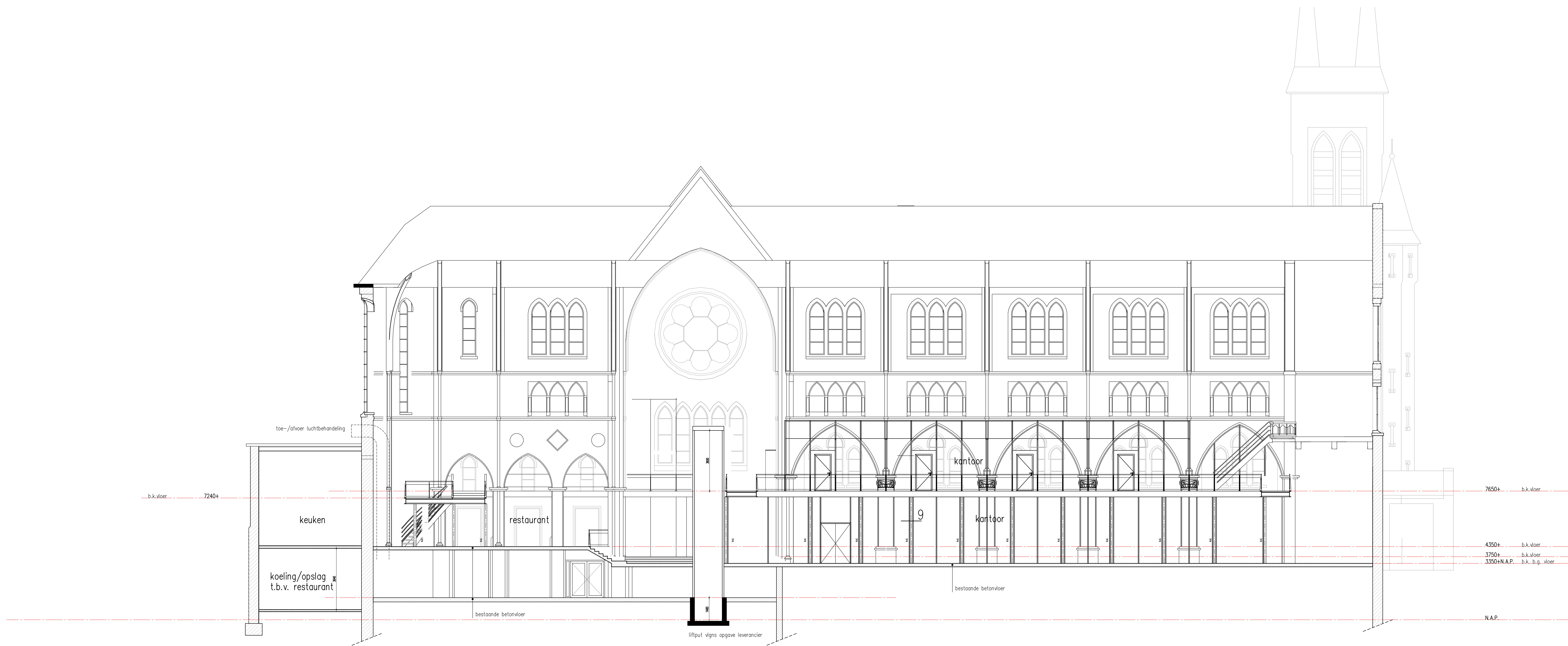
Doorsnede B-B
