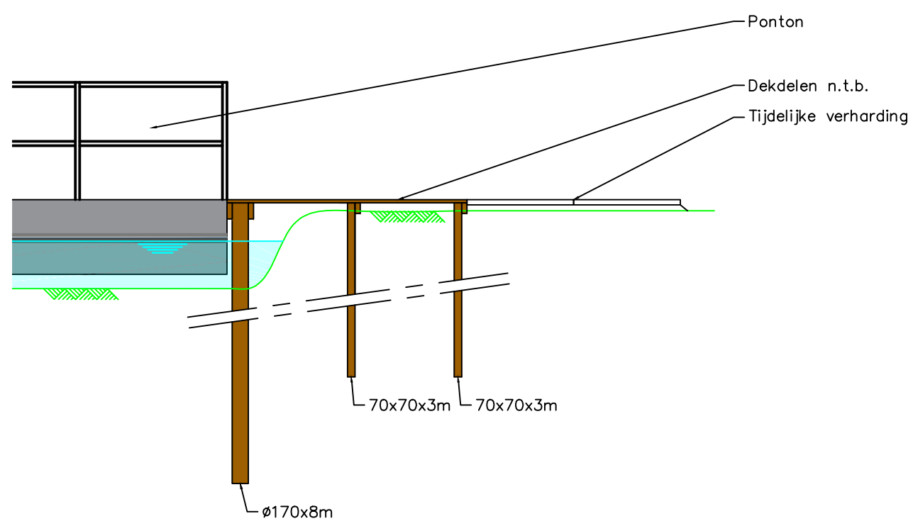
Steiger aanlandingsconstructie schaal 1:50
