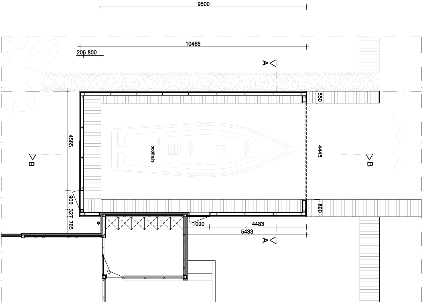
Begane grond
