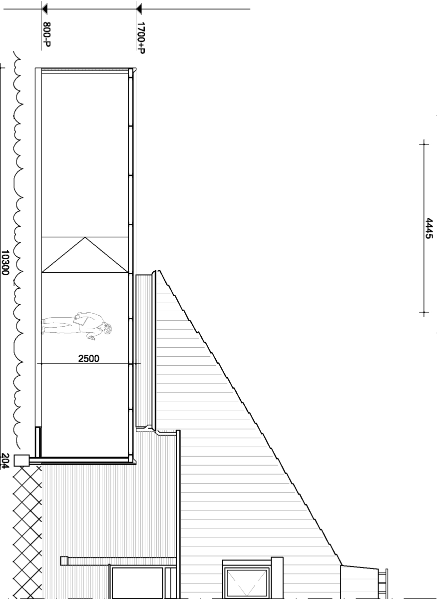
Doorsnede B-B
