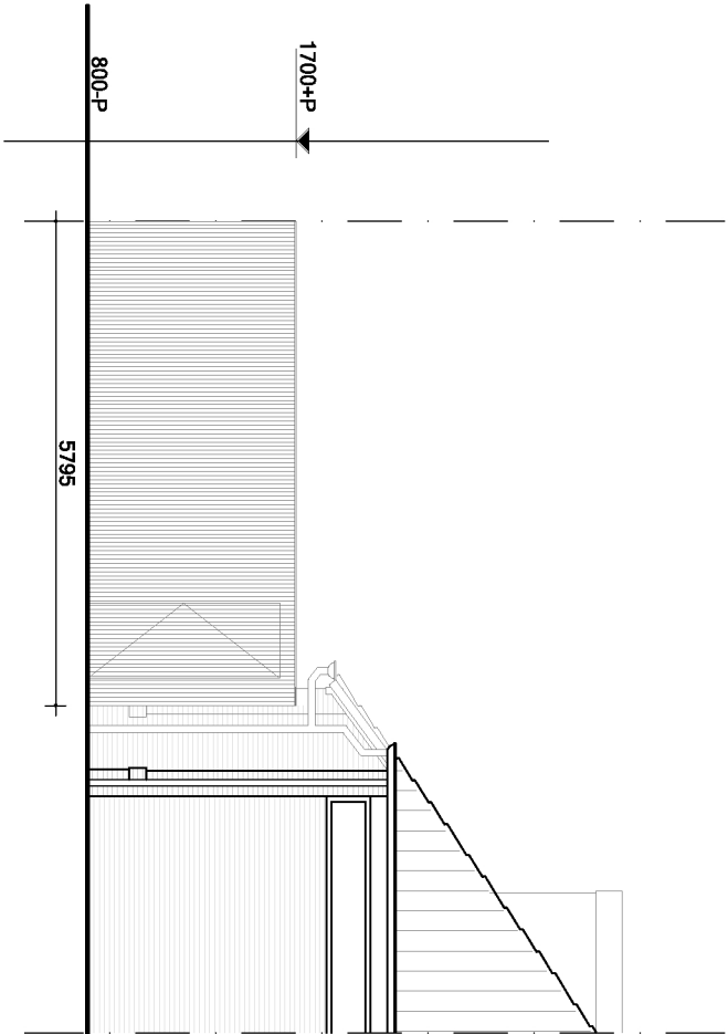
Voorgevel
