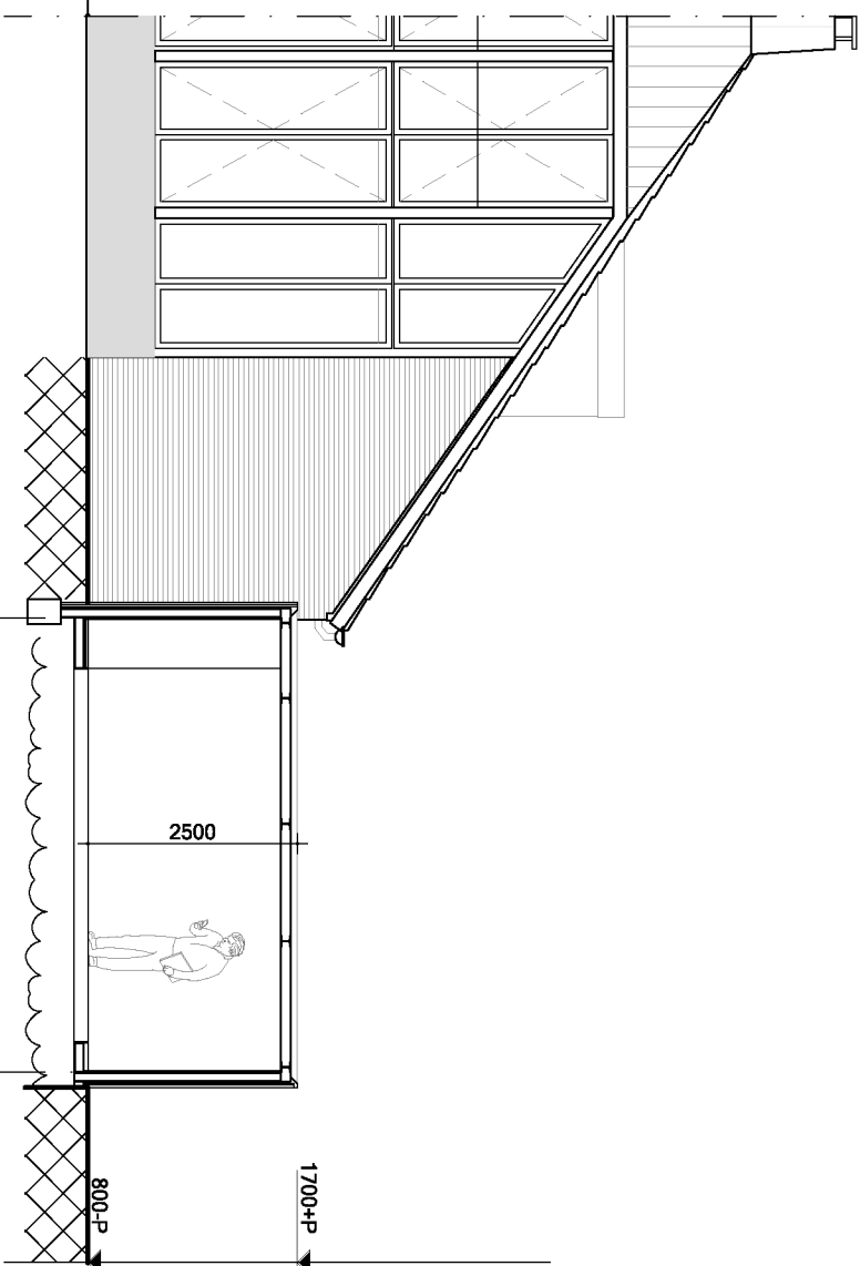
Doorsnede A-A + Achtergevel
