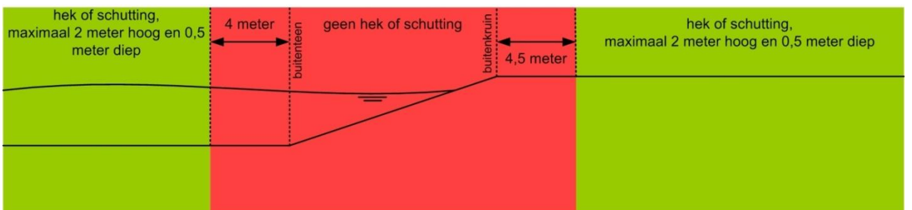
Figuur AR3.3: hek of schutting verheelde en aangeheelde waterkering
