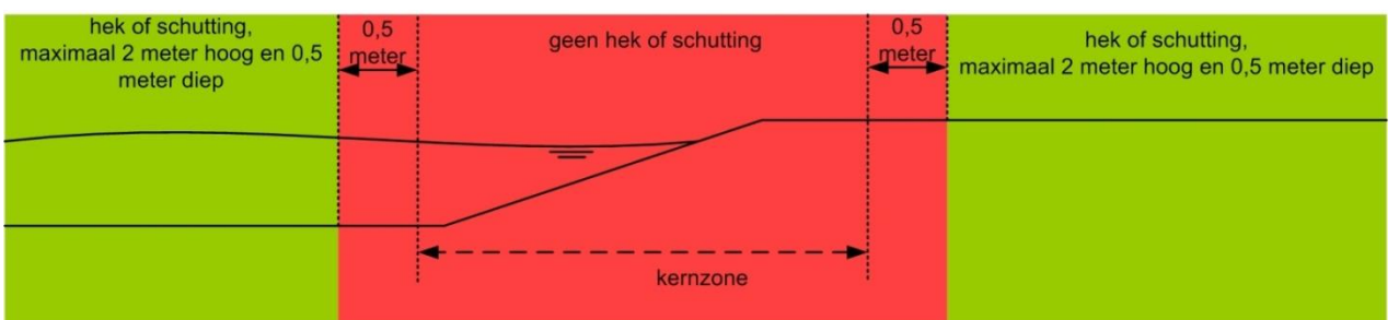
Figuur AR3.4: hek of schutting kadastrale erfafscheiding verheelde en aangeheelde waterkering
