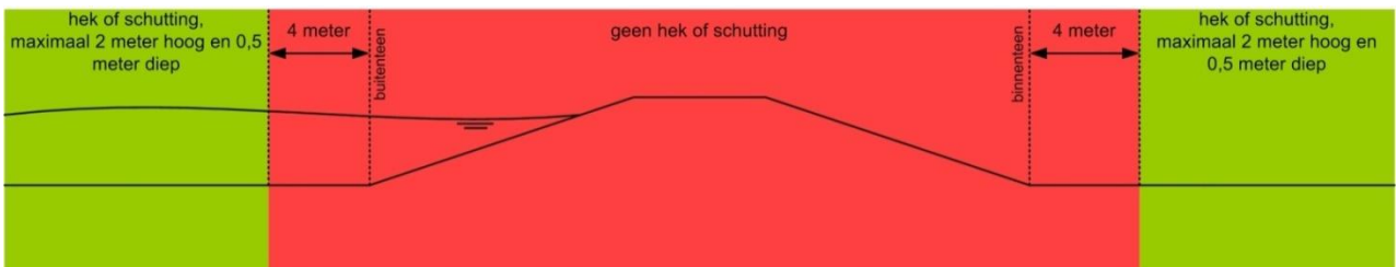
Figuur AR3.1: hek of schutting niet verheelde en niet aangeheelde waterkering
