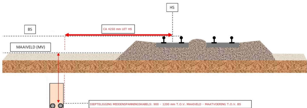
Figuur: Positionering netten; dekking en diepten
