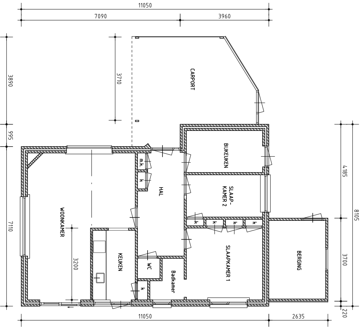
PLATTEGROND - BESTAAND 1:100
