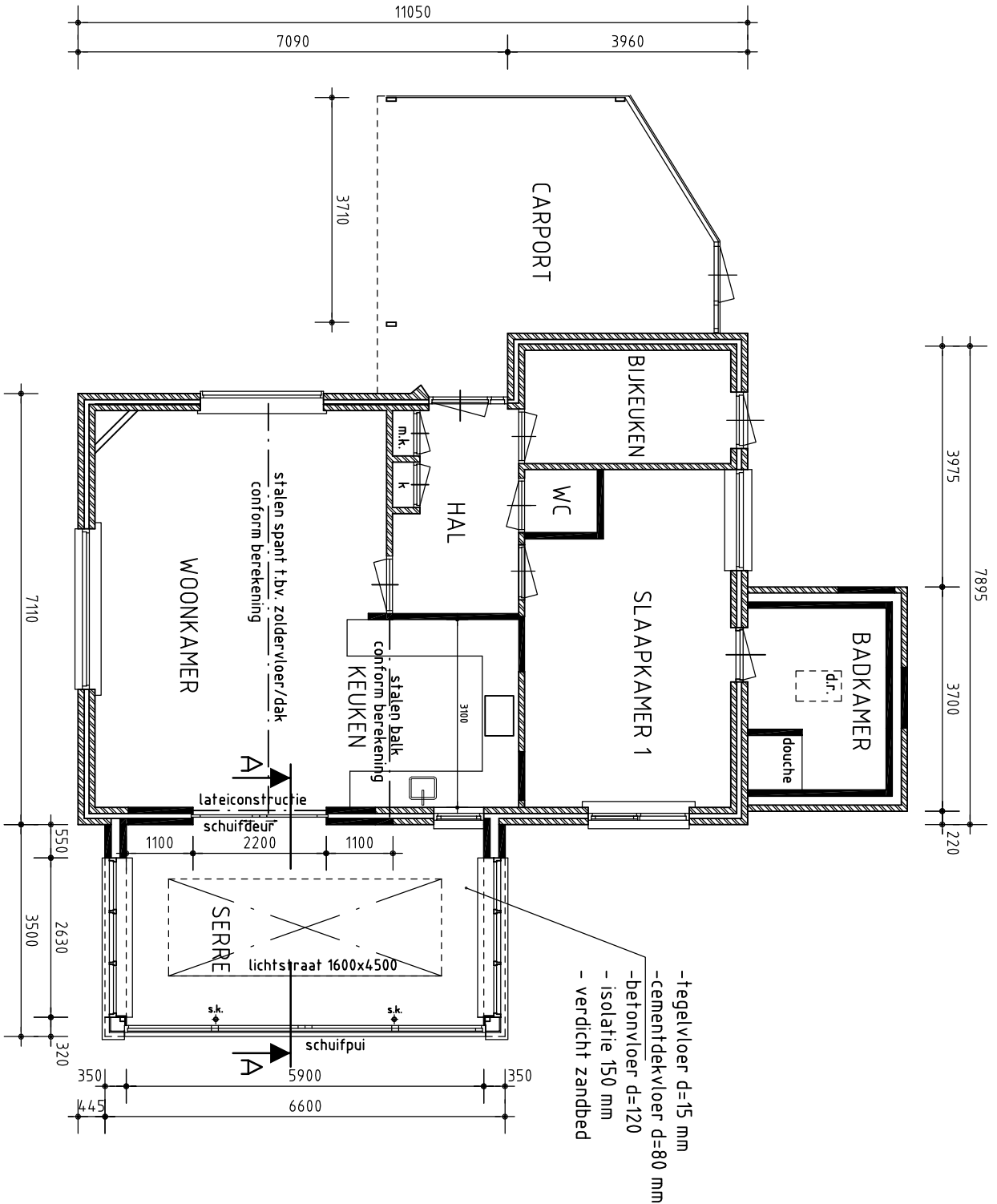
PLATTEGROND - NIEUW 1:100
