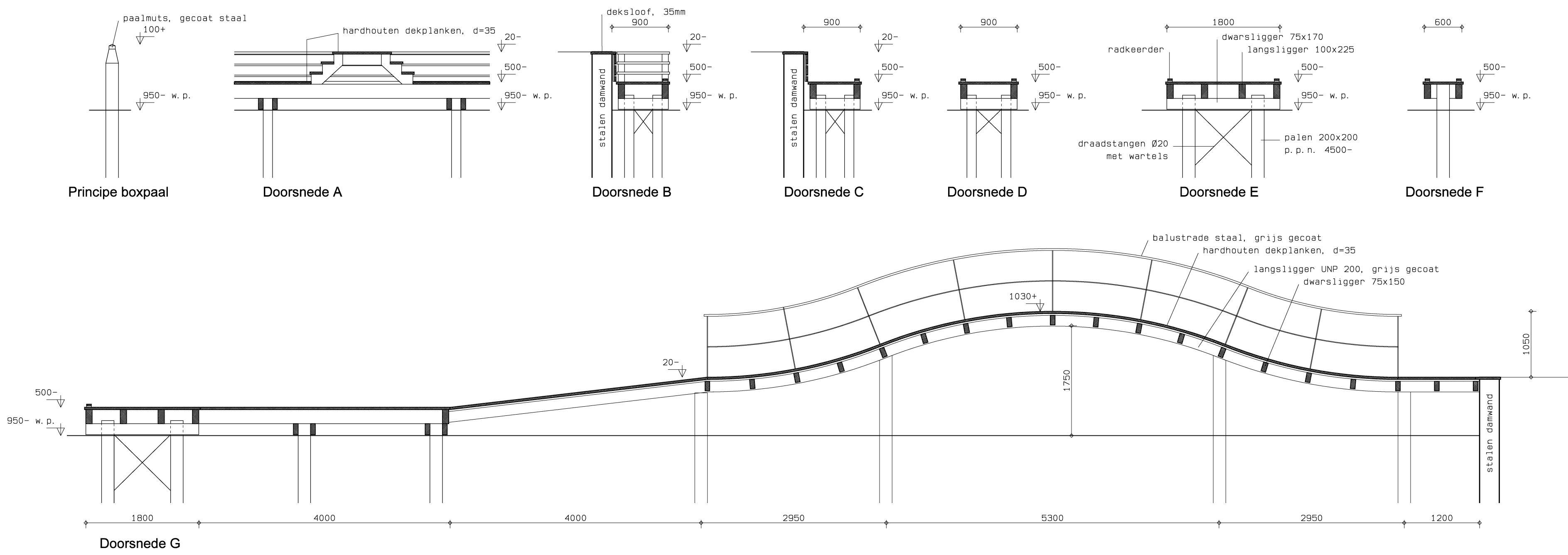
PRINCIPEDOORSNEDEN STEIGERS EN VLONDERS . 1:50
