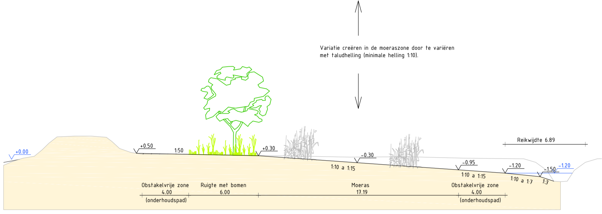
Profiel A Bestaand profiel conform profiel (d.d. 19-09-2012) schaal 1 : 200
