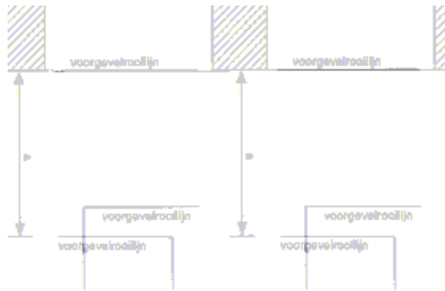
Figuur 16 Bouwhoogte in de voorgevelrooilijn (artikelen 2.5.20, vierde lid, tweede alinea)
