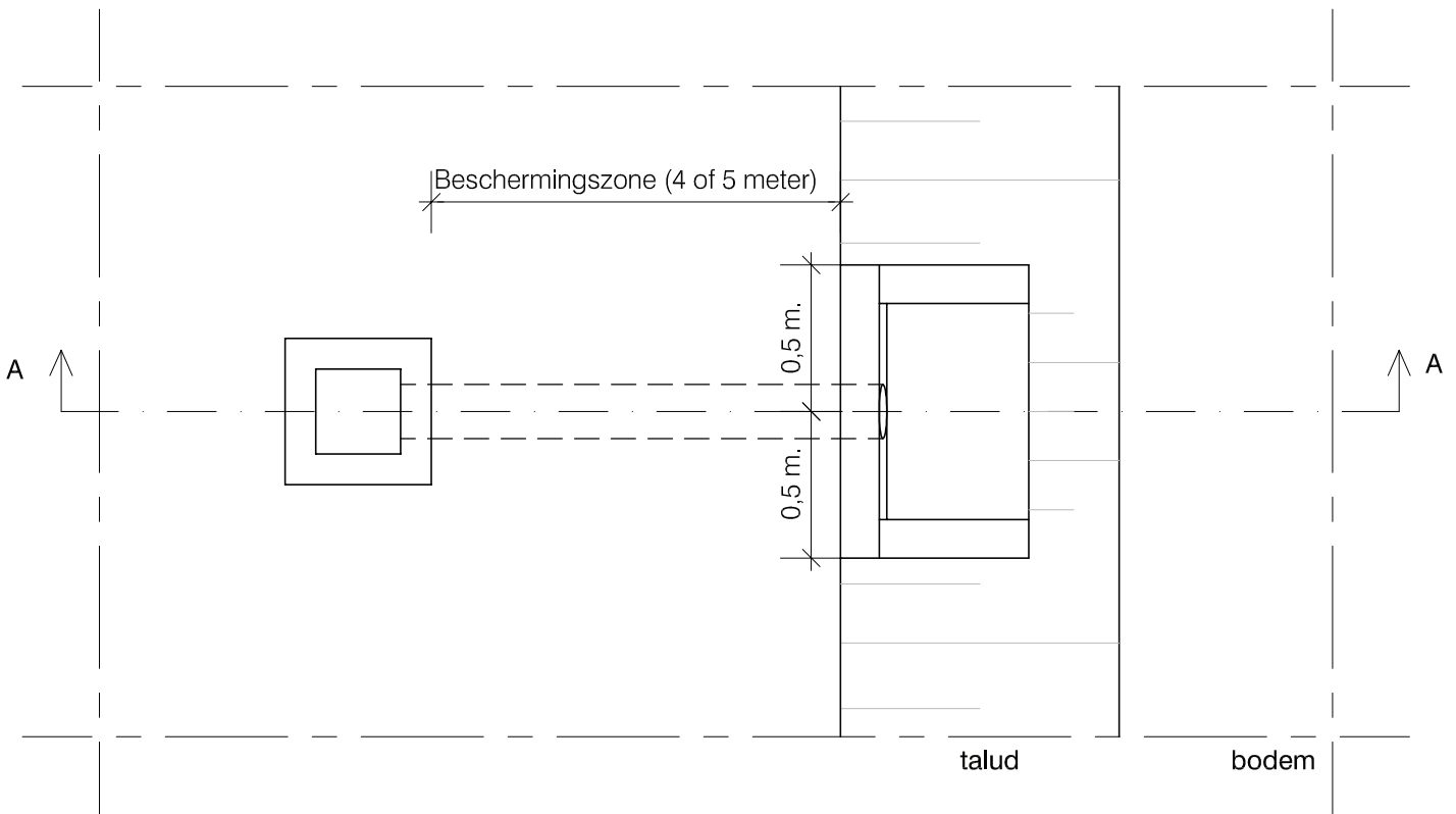
Bovenaanzicht
