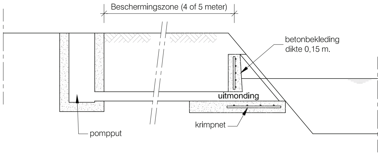
Dwarsdoorsnede A-A
