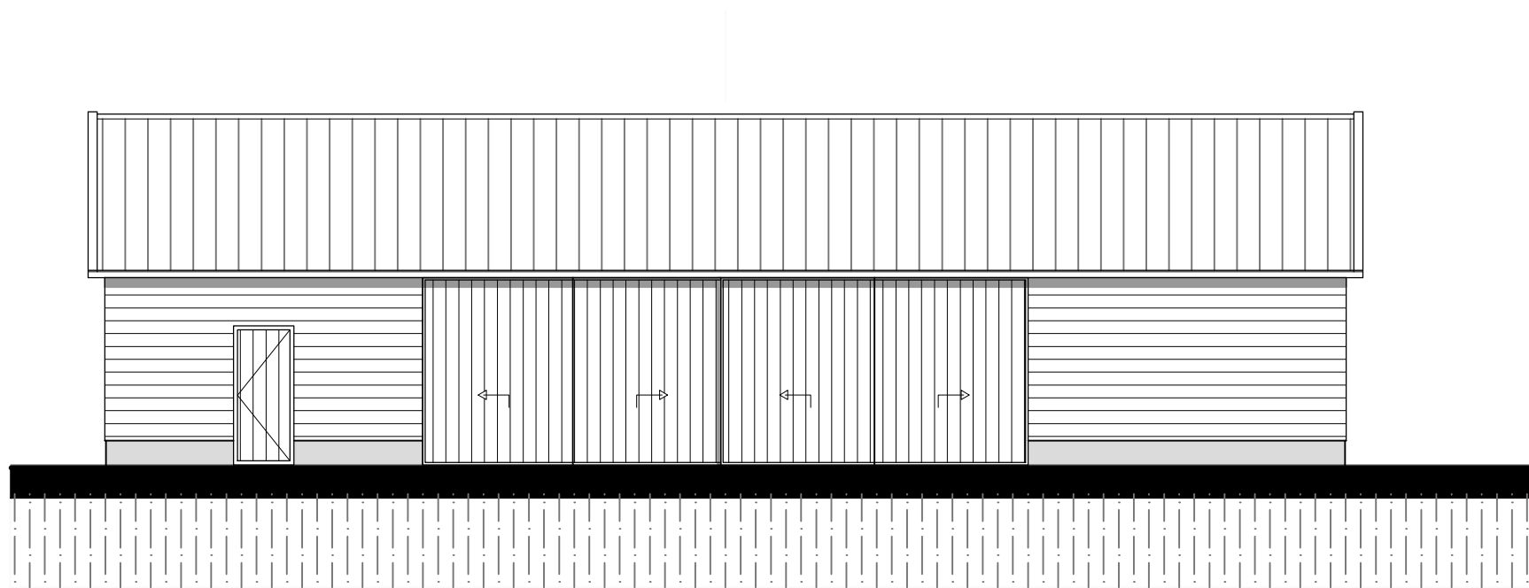
VOORGEVEL (ZUID)
