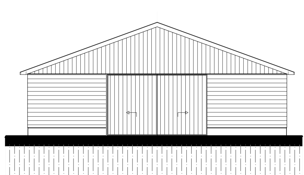
RECHTER ZIJGEVEL
