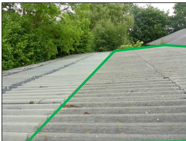
Foto 9: Schuur 1: Golfplaten dak (M03V)
