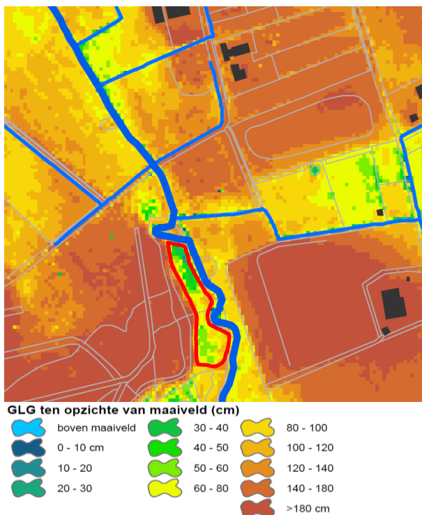
Figuur 5: Huidige situatie, gemiddeld laagste grondwaterstand ten opzichte van het Maaiveld (Bron: Valkenhorst scenario 5, Grondwatermodel Grootte Heide en Leenderbos)
