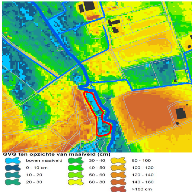
Figuur 4: Huidige situatie, gemiddelde voorjaarsgrondwaterstand ten opzichte van het Maaiveld (Bron: Valkenhorst scenario 5, Grondwatermodel Grootte Heide en Leenderbos)
