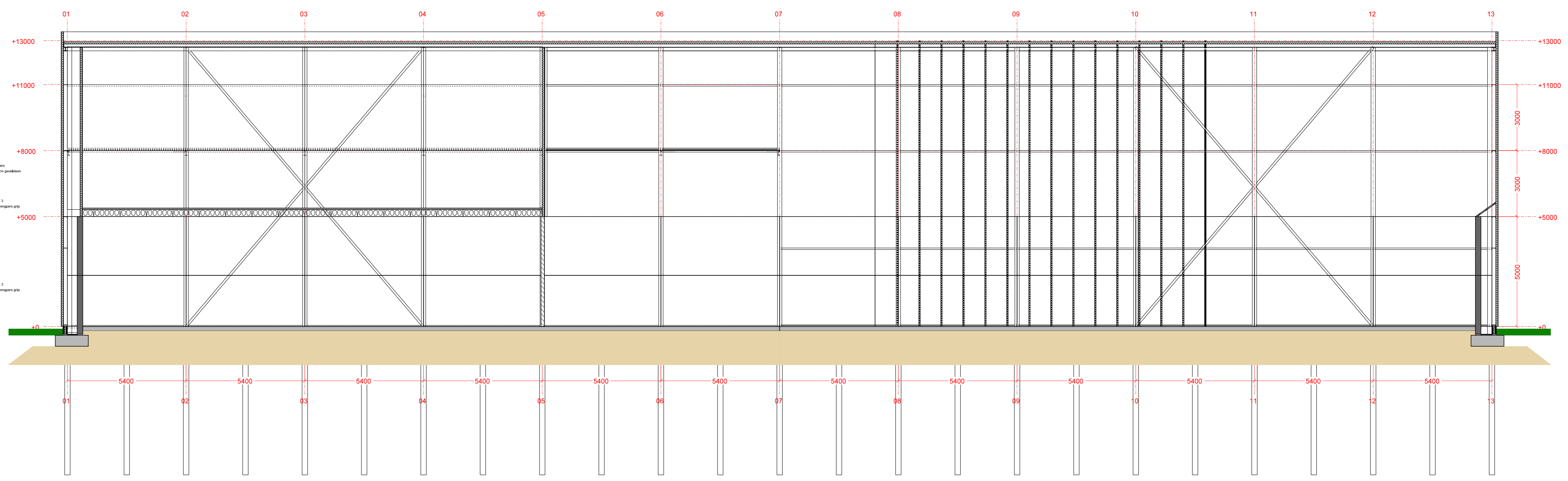
AANZICHT AS G 1:100
