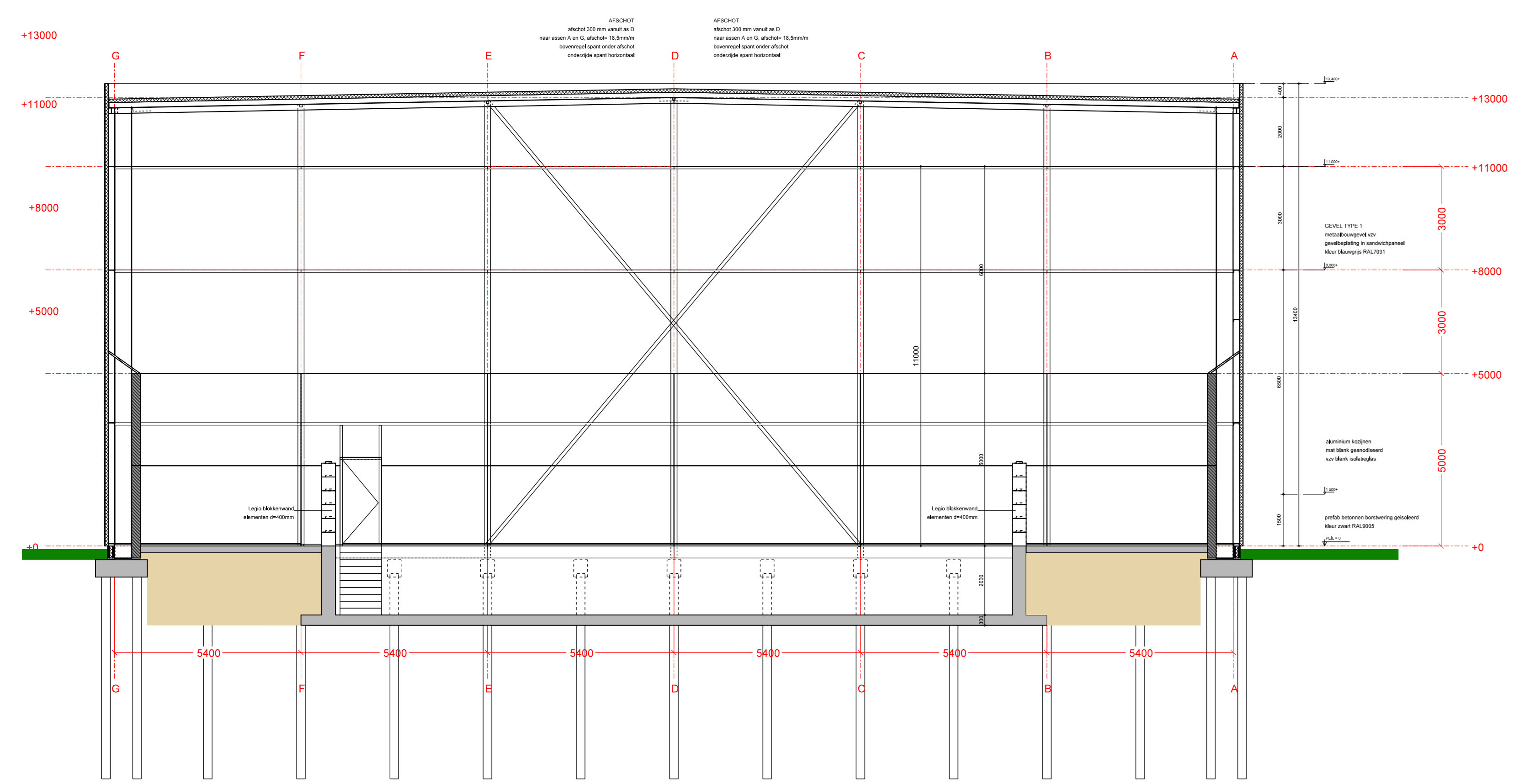
AANZICHT AS 13 1:100
