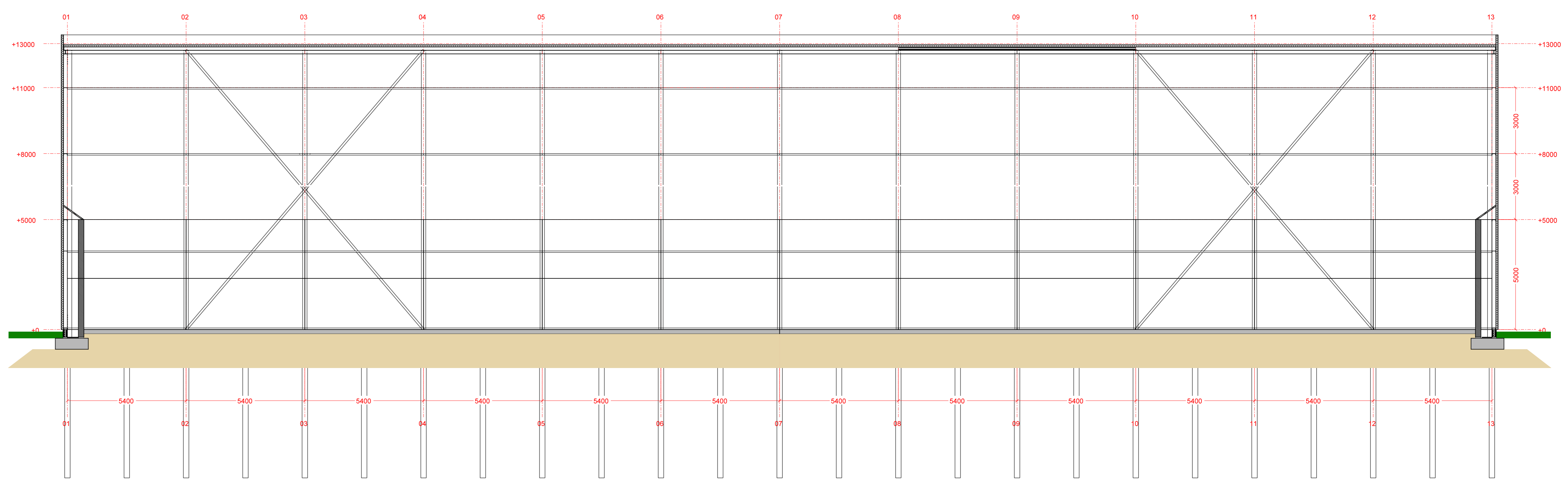
AANZICHT AS A 1:100
