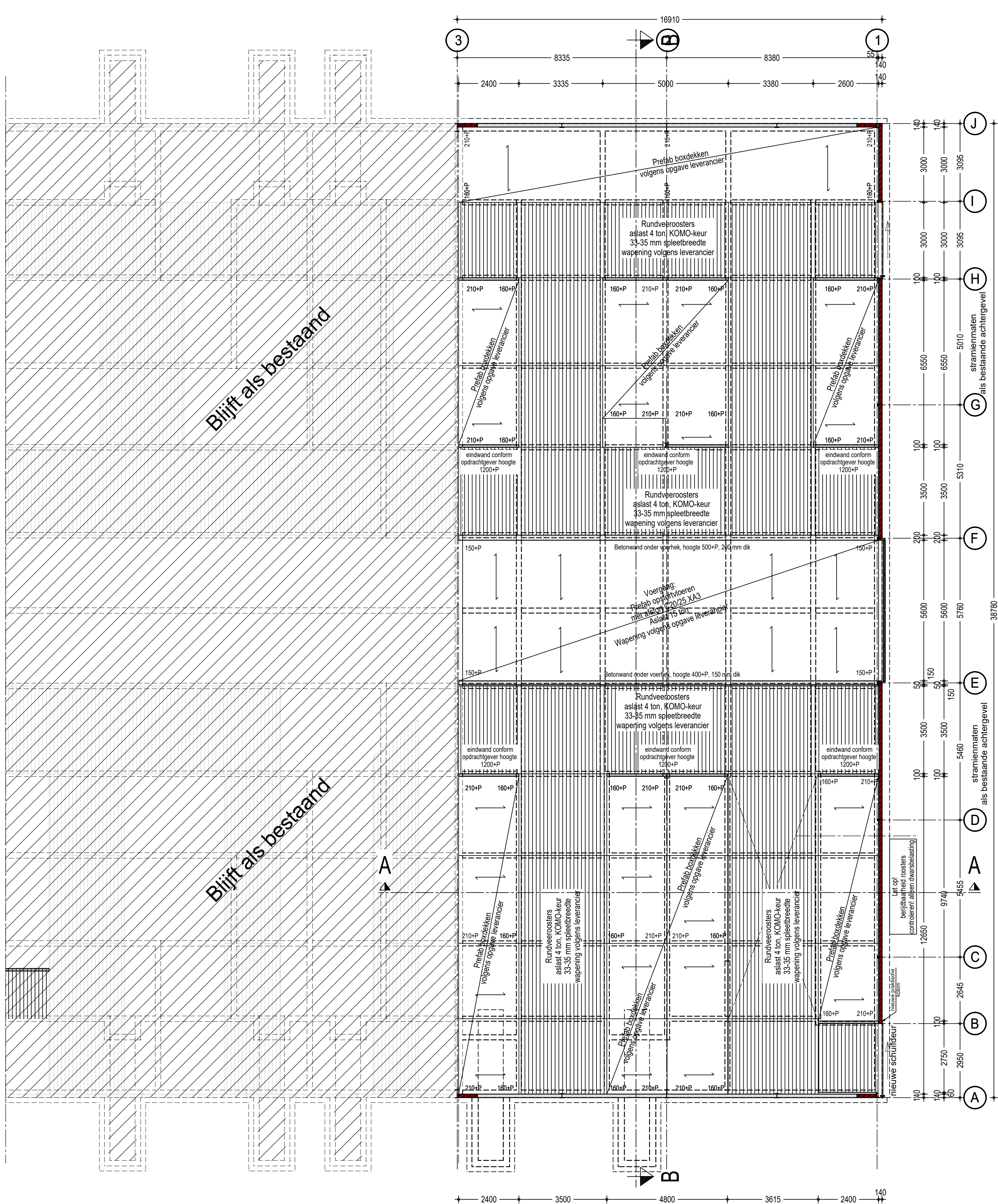
Vloerenplan
