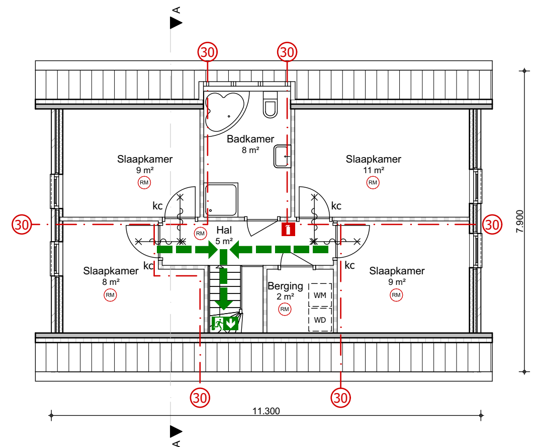
1e verdieping
