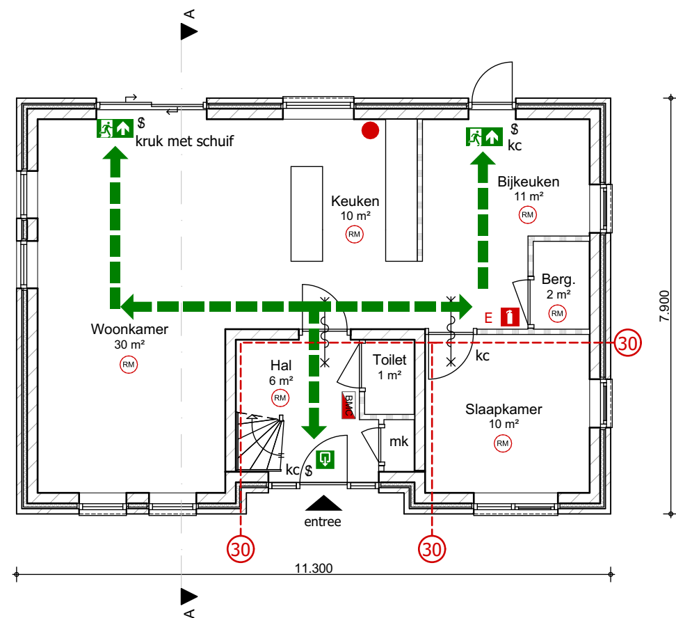
Begane grond
