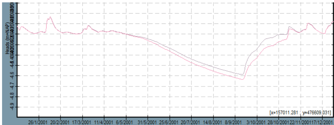
Figuur 3.8 Gemodelleerde tijd-grondwaterstandsgrafieken (blauw: aangepast, rood: oorspronkelijk)
