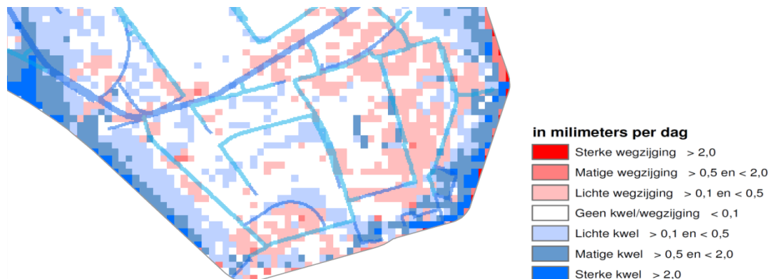
Figuur 2.16 Kwel en wegzijging (bron: AZURE)
