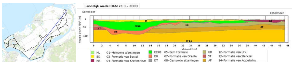
Figuur 6 Geohydrologische dwarsdoorsnede
